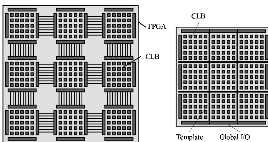
(a) Multi-FPGA con topología de malla (b) Modelo SFGPA
