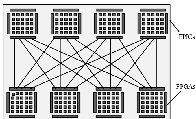
Figura 2.6 Topología de Barras Cruzadas
