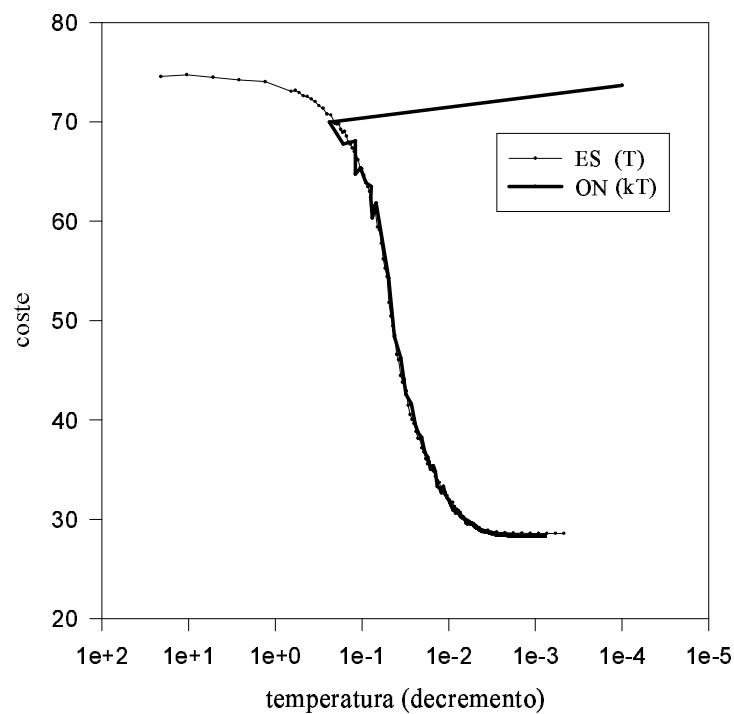
Figura 3.4 Evolución de la relación coste/temperatura para las ubicaciones con ES y ON
