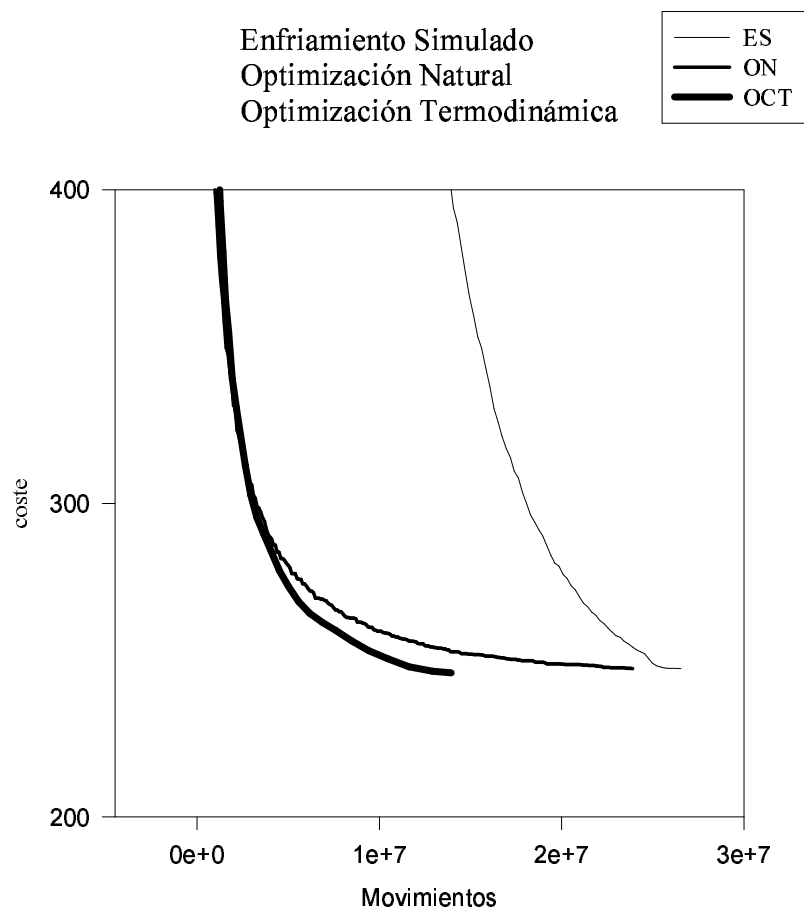
Figura 4.1 Comparación de la evolución coste/movimientos para la optimización con ES , ON y OCT en el problema de la ubicación sobre FPGAs.
