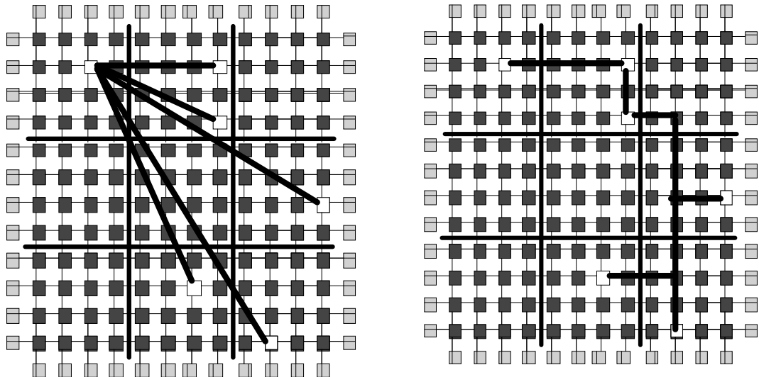
(a) Indeterminación del cableado (posible conjunto de corte para una red multiterminal)
