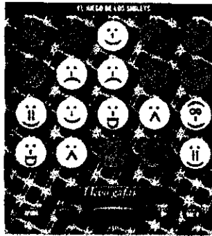
Shockwave (137K)
