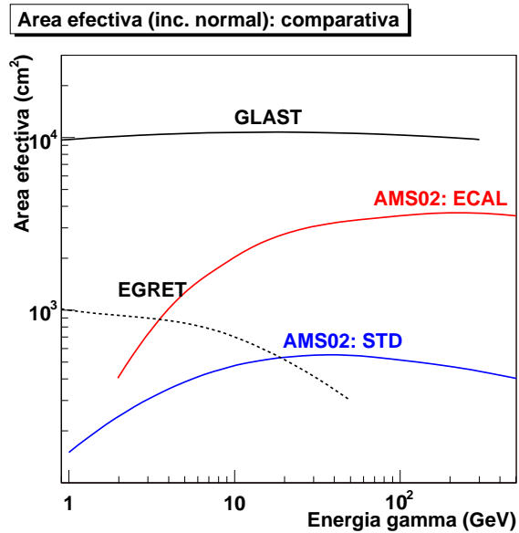
Figura 3.26: Comparativa de área efectiva en incidencia normal en función de la energía.
