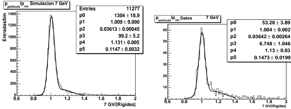
Figura 4.30: Distribución de p_{haz}/p_{rec} para 7 GeV en simulación y datos. Sobreimpuesto un ajuste a 2 Gaussianas.
