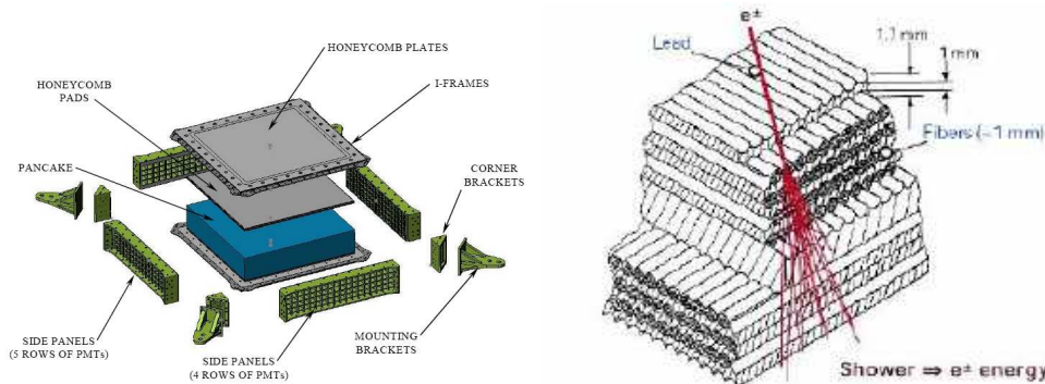
Figura 2.13: Vista explosionada del calorímetro electromagnético de AMS-02 con el volumen de detección (pancake) rodeado de las estructuras de soporte (izquierda). A la derecha, se muestra un corte de la estructura interna del pancake donde es visible la disposición cruzada de las fibras de centelleador y el volumen pasivo de plomo.
