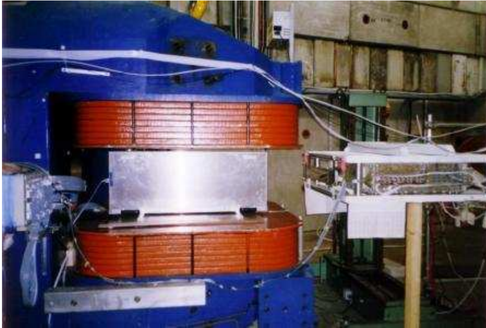
Figura 4.6: Detectores STD2, STD3 y ECALD. Vista lateral.
