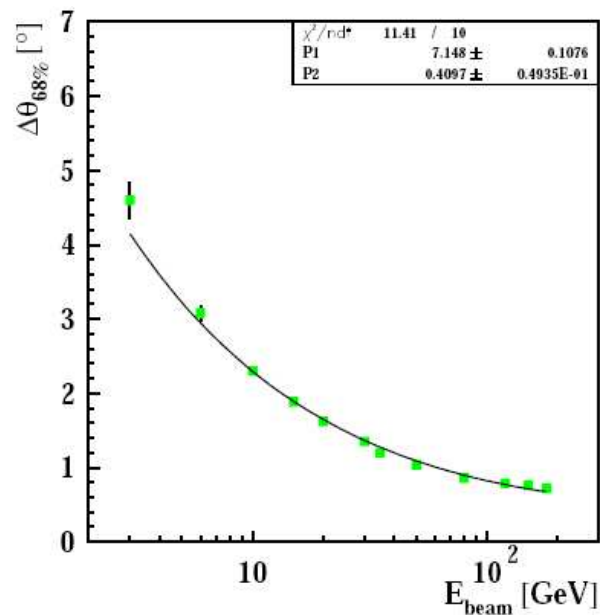
Figura 3.24: Resolución angular en función de la energía: ECAL [3].
