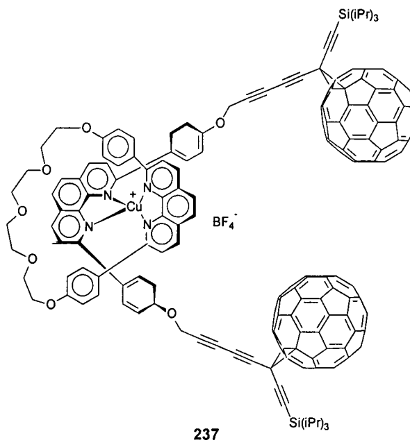
Figura 111. Estructura del rotaxano 237 con aplicaciones en la construcción de arquitecturas moleculares.
