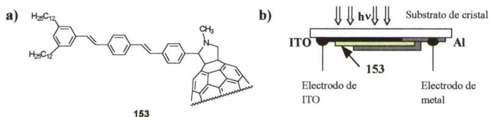
Figura 62. a) Estructura de la díada 153 ; b) Diseño de una célula fotovoltaica en la que se encuentra incluida la nueva díada.
