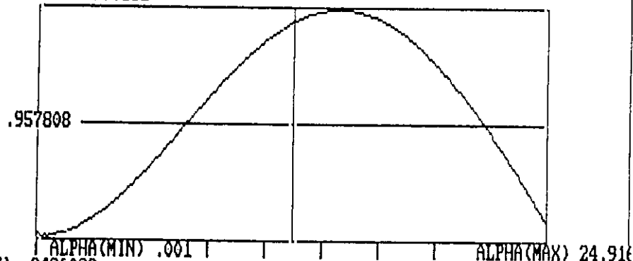
Fig.A.4.1. (1)Detalle de salida del código 1-(MCARSI) Aluminio sin compensar con módulo elástico. (2) Intervalos de confianza resultados código 1. (aluminio sin compensar con m.e.) (3) Tabla del ANOVA resultados código 1.(aluminio s.c.m.e.).(4). Detalle del recorrido del coeficiente R, en relación con la variación de \alpha .
