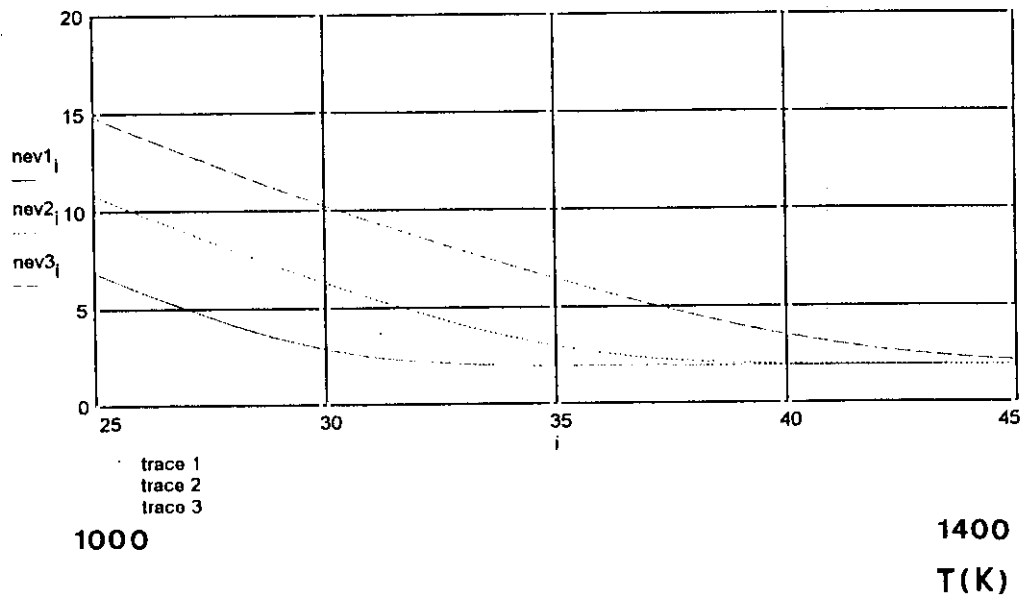
Fgi.A6.14. Representación de la variación del valor de n_{\text{efectivo}} , con la temperatura para tres valores de la velocidad de deformación: 1) v=0.0025 \text{ seg}^{-1} , 2) v=0.135 \text{ seg}^{-1} , 3) v=7.38 \text{ seg}^{-1} . Para una velocidad de deformación dada, n , disminuye con la temperatura, quedando los valores de n , dentro de una cierta constancia, o al menos pequeña variabilidad, en el rango de Temperaturas entre 1200 y 1400 K tendiendo los valores de n a un valor asintótico mínimo n=1.96 , que es el valor de ajuste de la ecuación de Garofalo.
