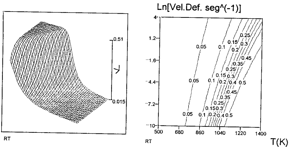
Fig.A.6.5. Representación tridimensional de la eficiencia total \eta = J/G = RT . Mapa de líneas de nivel. Isolineas son líneas de igual valor para \eta
