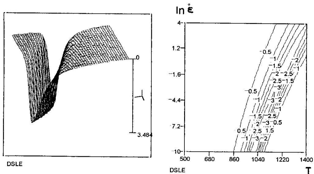
Fig. A.6.8. Representación de L1(T, \dot{\epsilon}) = \frac{\partial m}{\partial \ln(\dot{\epsilon})} , frente a la temperatura y a la velocidad de deformación. Mapa de isolineas. Las curvas de nivel son curvas de igual valor de L1.
