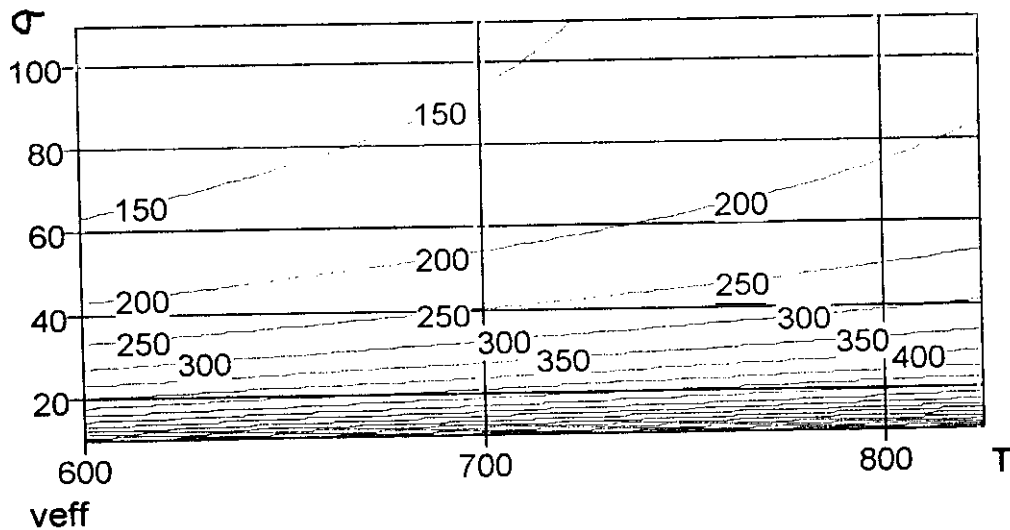
Fig.A.6.56. Representación tridimensional de V_{\text{efectivo}}=V_e frente a la tensión y temperatura de trabajo. Representación del mapa de isolineas correspondiente. Líneas de igual nivel son líneas de V_e=\text{constante}
