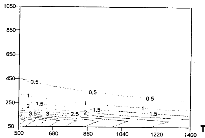
Fig.A.6.11. Representación del factor L2(\sigma, T) = \frac{\partial \sigma}{\partial \ln(\dot{\epsilon})}(T, \sigma) , frente a la tensión y la temperatura. El mapa de isolíneas representa las curvas de nivel de igual valor de L2
