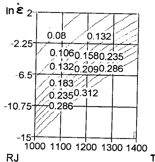
Fig.A6.23. Representación tridimensional del factor de eficiencia \eta_J , frente a la velocidad de deformación y la temperatura. Representación correspondiente del mapa de isocurvas. Curvas de igual nivel representan \eta_J = \text{constante} .
