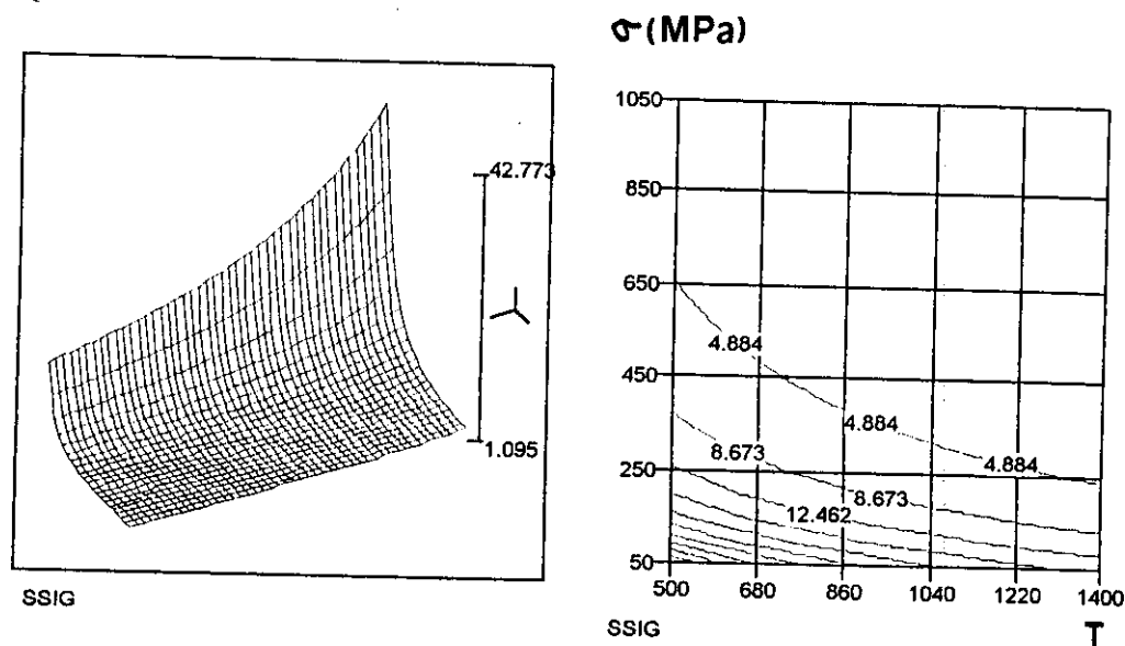
Fig. A.6.7 Coeficiente de entropía diferencial del sistema, frente a la temperatura y a la tensión. Mapa de curvas de nivel. Isolineas corresponden a las curvas de igual valor del coeficiente diferencial de entropía.
