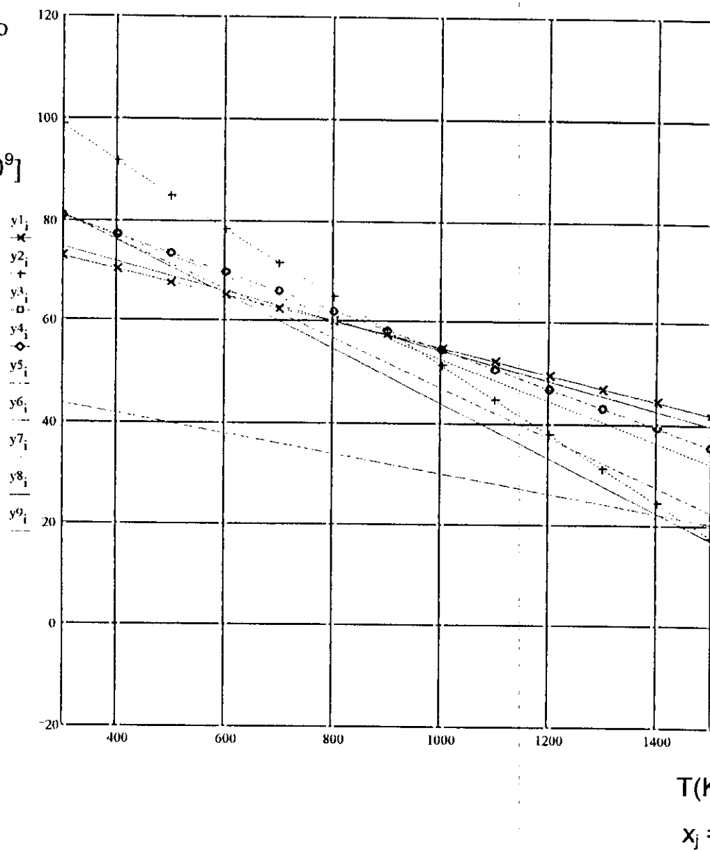
Fig.A5.12. Representación de la colección de módulos de cizalla para diferentes aceros ( los mismos que los de la figura A5.11)
