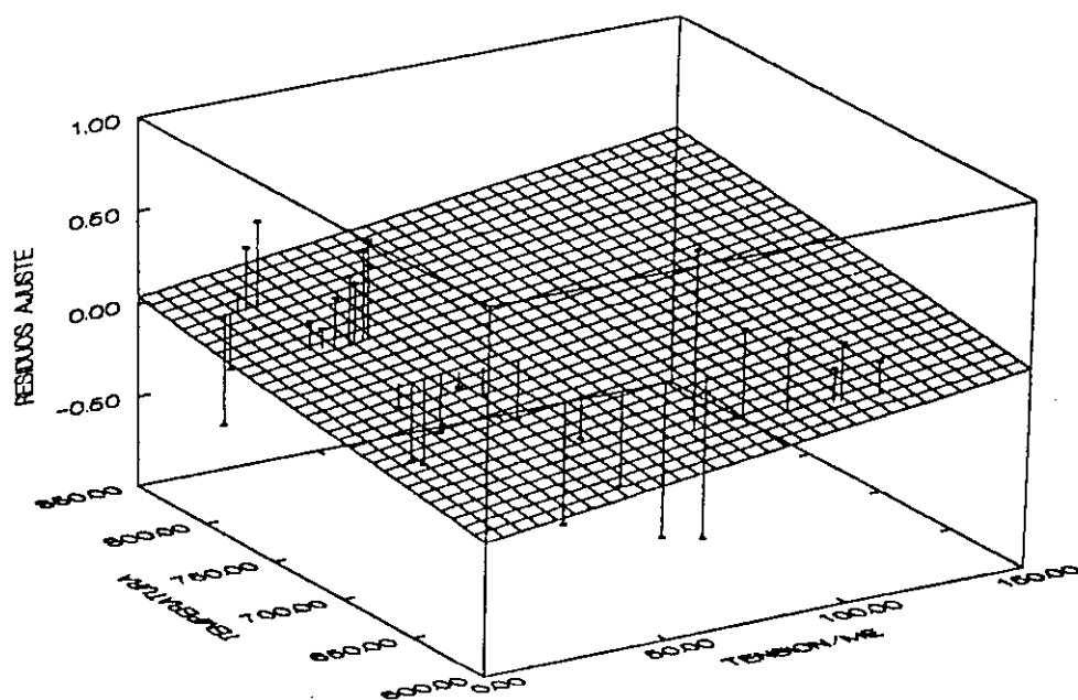
Fig.(58). Representación tridimensional de los residuos del ajuste de la ecuación de Garofalo a los datos de aleación de aluminio, frente a \sigma/E , y temperatura (K). Se representa el plano de regresión promedio de los residuos.
