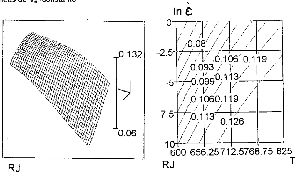
Fig.A.6.56. Representación tridimensional de V_{\text{efectivo}}=V_e frente a la tensión y temperatura de trabajo. Representación del mapa de isolineas correspondiente. Líneas de igual nivel son líneas de V_e=\text{constante}
