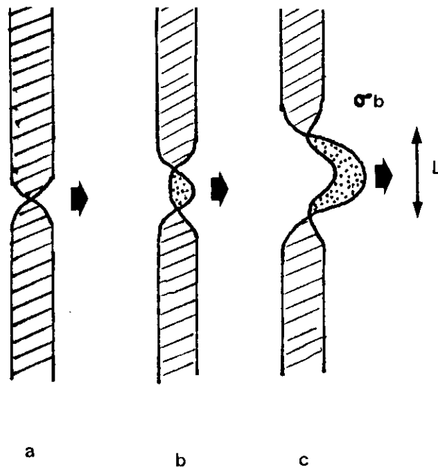
Fig.(92). Deslizamiento cruzado de una dislocación en arita. La contracción de la banda de falta de apilamiento (a) se desarrolla en (b) dividiéndose en el plano de deslizamiento cruzado, al ensancharse la división por acción de la tensión conductora del proceso (c).
