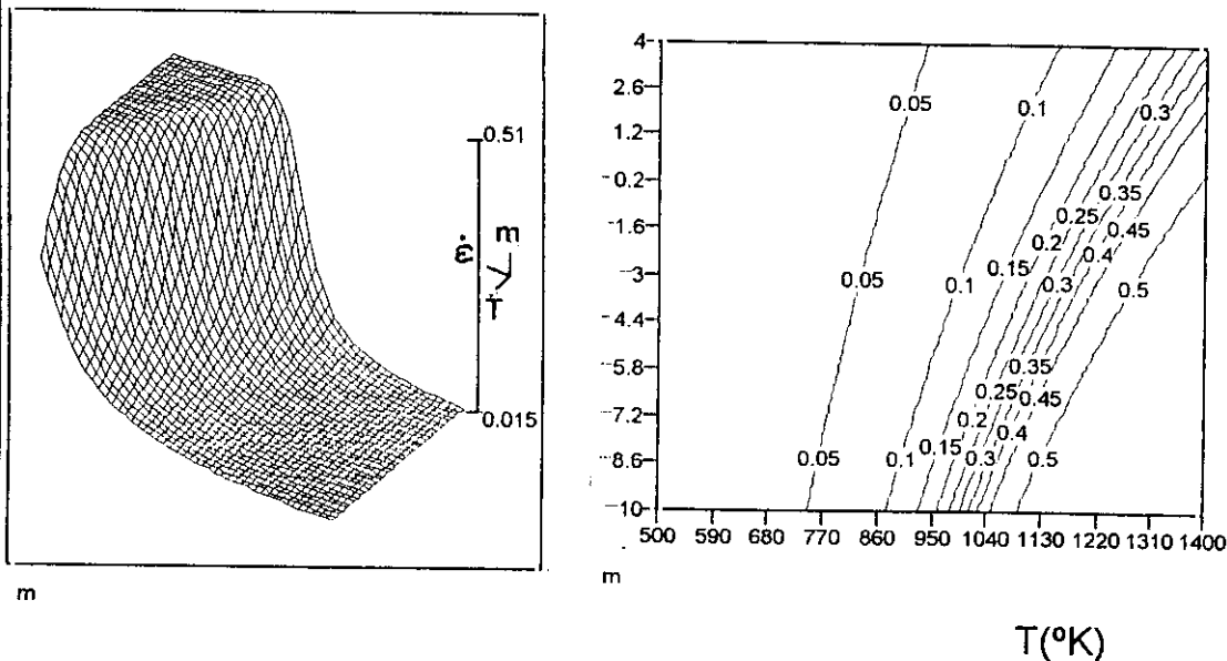
Fig.A6.1 Representación tridimensional de m , frente a Temperatura y logaritmo de las velocidades de deformación. Mapa de curvas de nivel de igual valor de m . Las isolneas son líneas de valor igual de m .
