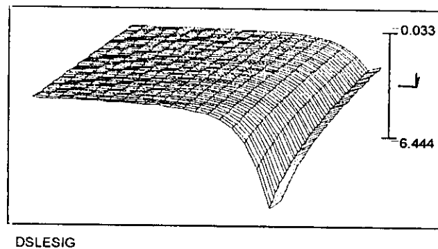
Fig.A.6.10. Representación de L1(\sigma) = \frac{\partial m}{\partial \ln(\dot{\epsilon})}(\sigma) , frente a la tensión
