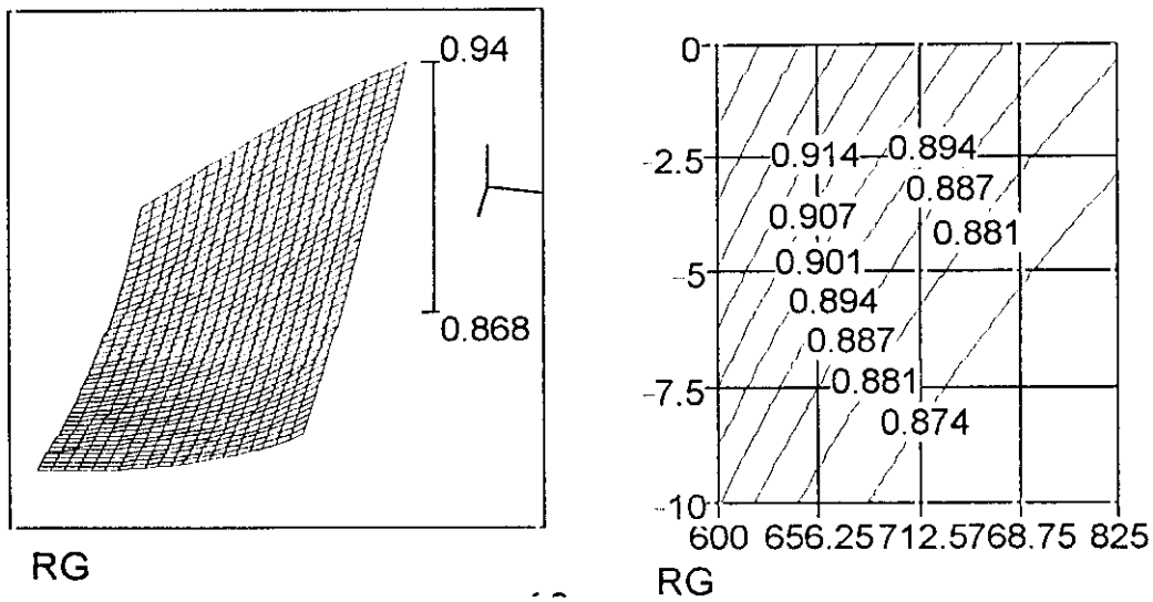
Fig.A.6.59. Representación tridimensional del rendimiento del factor G , \eta_G frente a la temperatura y a la velocidad de deformación, con el correspondiente mapa de isocurvas. Las curvas de nivel representan el factor \eta_G = \text{constante} .
