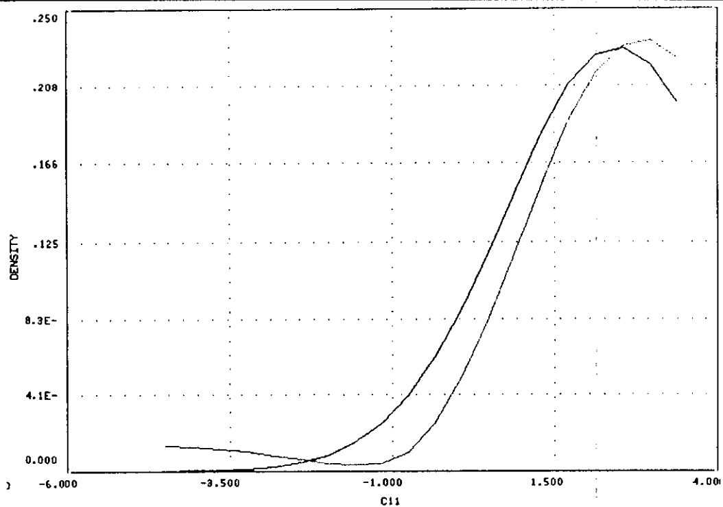
GRÁFICA 11. Representación de la función de densidad de la variable \ln(\epsilon'_{\max})
