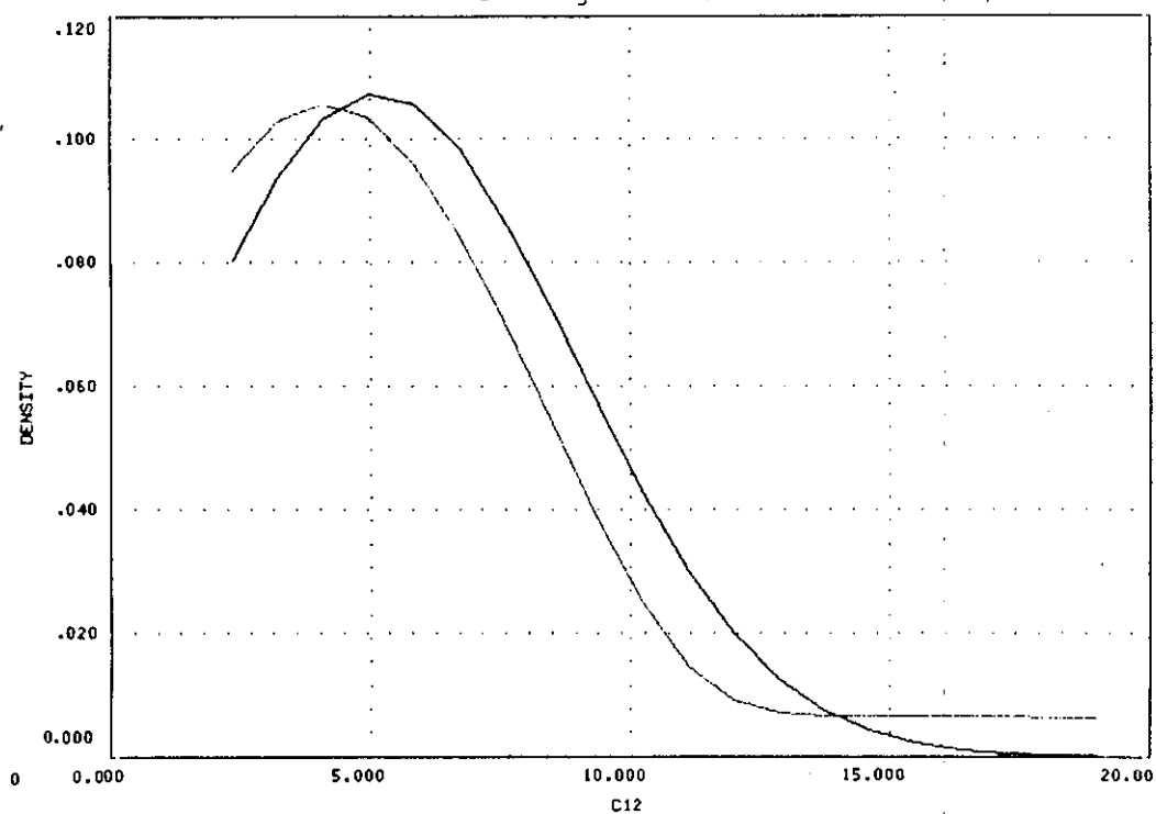
GRÁFICA 12. Representación de la función de densidad de la variable \ln(r'_{\max}/r'_{\min})
