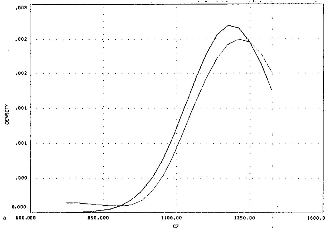
GRÁFICA 7. Representación de la función de densidad de la variable T_m
