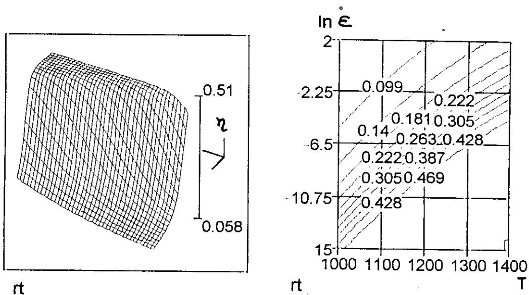
Fig.A.6.25. Representación tridimensional del rendimiento del factor G , \eta_G frente a la temperatura y a la velocidad de deformación, con el correspondiente mapa de isolneas. Las curvas de nivel representan el factor \eta_G = \text{constante} .
