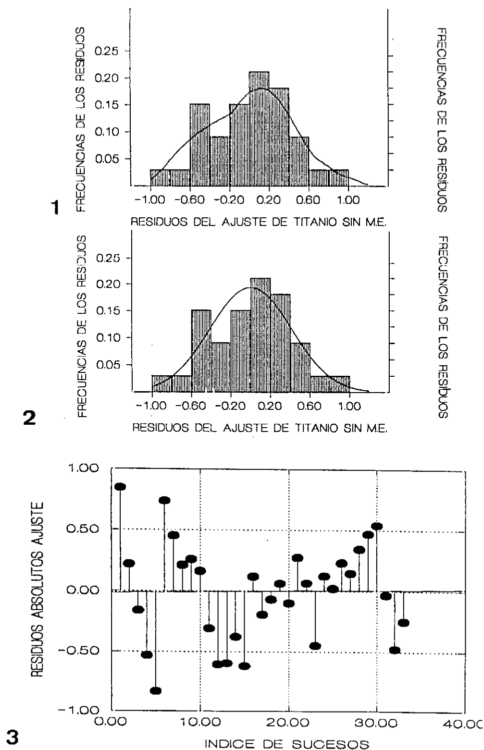
Fig.A.4.15. (1) Representación de la función de frecuencia de los residuos cuando los controles de convergencia han sido muy restrictivos en el código 2, y cuando la maya de seriación del código 1, ha sido muy fina. (2) Ajuste de la mejor función de distribución normal a los residuos del ajuste. Titanio sin compensar las tensiones con el módulo elástico.(3). Seriación de los residuos del ajuste.
