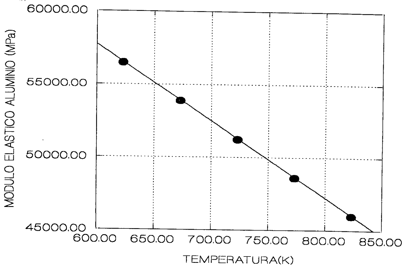
Fig.A5.1 Módulo elástico utilizado para el ajuste de la aleación de Aluminio
