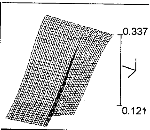
Fig.A.6.24. Representación tridimensional del factor de eficiencia \eta_J , frente a la tensión y la temperatura. Representación correspondiente del mapa de isocurvas. Curvas de igual nivel representan \eta_J = \text{constante} .
