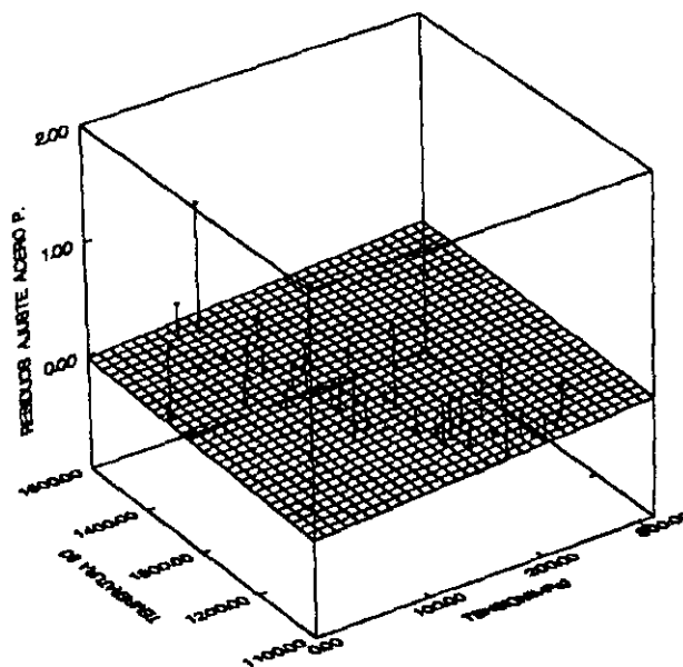
Fig.(37). Representación tridimensional de los residuos del ajuste del acero A2, respecto de la tensión (Mpa) y la temperatura (K), con el plano de regresión ajustado para los residuos
