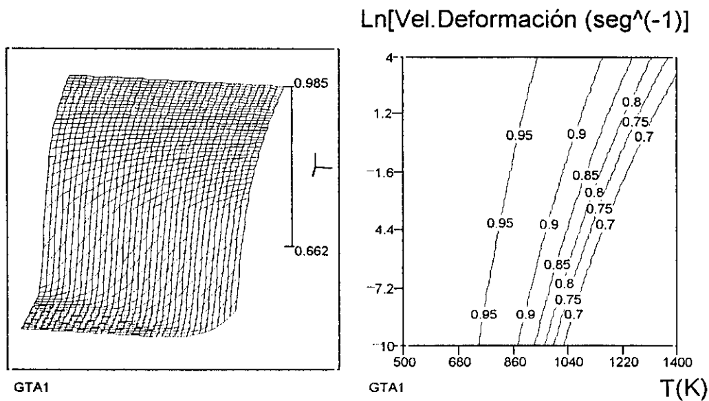
Fig.A.6.4. Representación del factor de eficiencia \eta_G = 1 - \eta_J , frente a la temperatura y a la velocidad de deformación. Mapa de curvas de nivel. Isolineas son las líneas de igual valor para la eficiencia \eta_G
