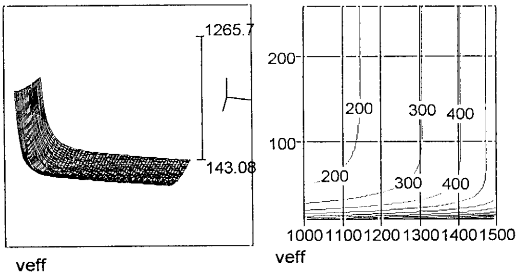
Fig.A.6.37. Representación tridimensional de V_{efectivo}=V_e frente a la tensión y temperatura de trabajo. Representación del mapa de isocurvas correspondiente. Líneas de igual nivel son líneas de V_e=\text{constante}
