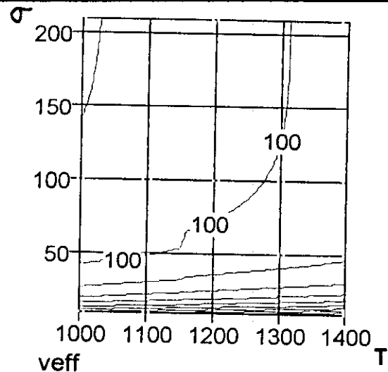
Fig.A.6.22. Representación tridimensional de V_{\text{efectivo}}=V_e frente a la tensión y temperatura de trabajo. Representación del mapa de isocurvas correspondiente. Líneas de igual nivel son líneas de V_e=\text{constante}
