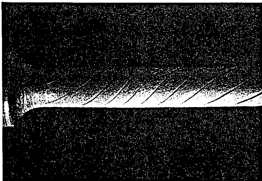
Fig.(11) Detalle de una probeta sometida a torsión con la producción de marcas previas que permiten valorar la forma de producirse la deformación
