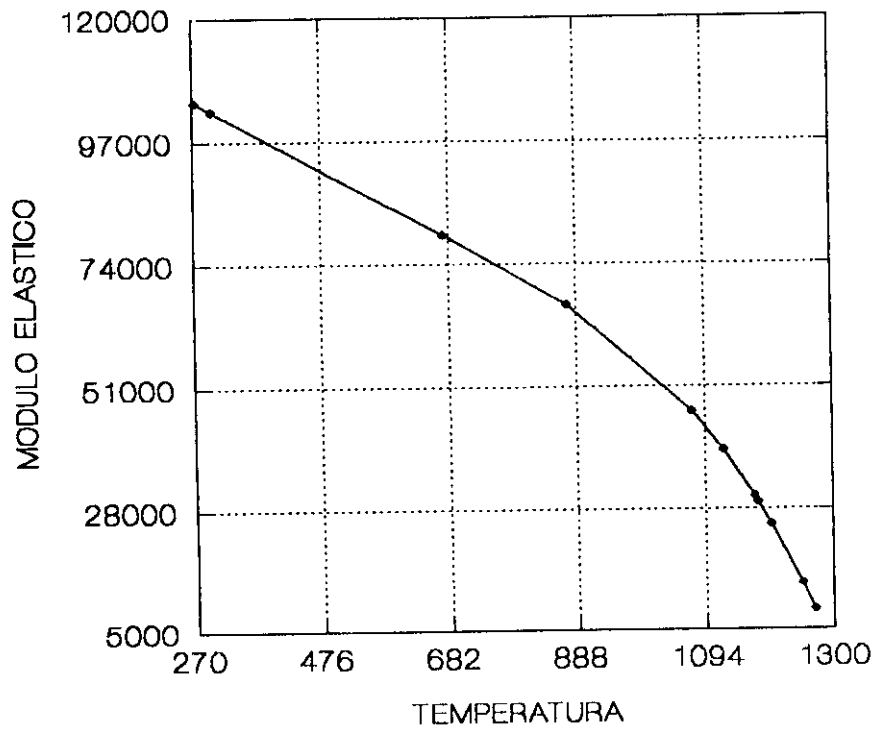
Fig.A5.3. Módulo de elasticidad (Mpa), frente a la Temperatura (K). Caso WK.
