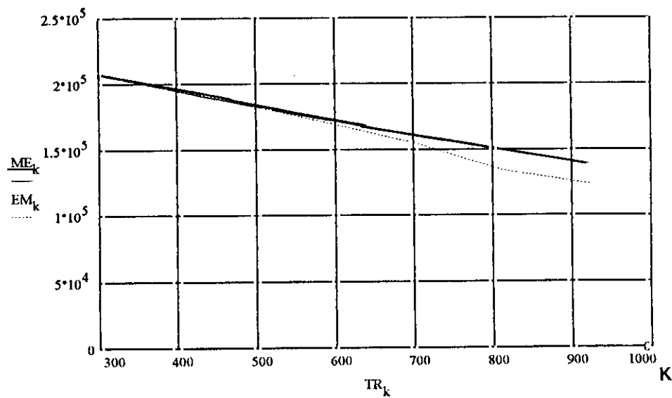
Fig.(70). Comparación de los datos experimentales del módulo elástico para aceros con contenido medio en carbono ( línea discontinua) frente a la función del módulo elástico calculada por métodos teóricos entre 300K y 1000 K. (línea continua)
