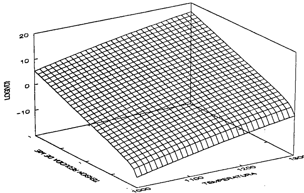
Fig.(52). Representación de la mejor superficie del ajuste de los datos experimentales de la aleación de titanio con las tensiones compensadas por el módulo elástico. \ln(\epsilon') , respecto de \sigma/E , y T(K) .
