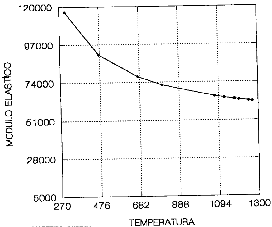
Fig.A5.4 Módulo de elasticidad (Mpa) frente a la Temperatura (K). Usado para el ajuste de la aleación de Titanio, no se adapta bien.
