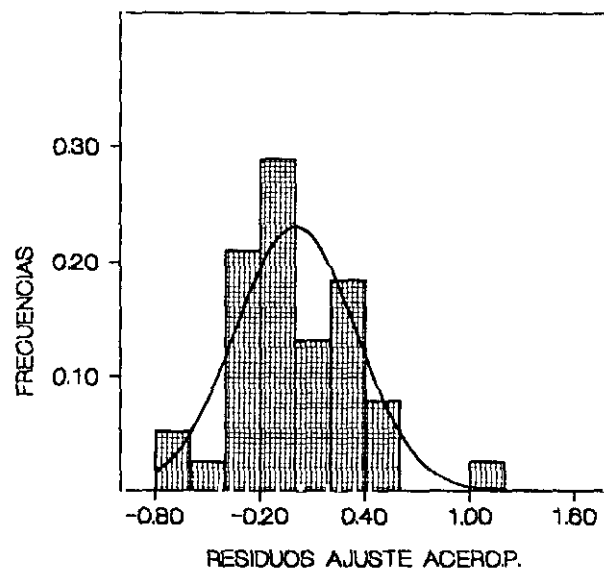
Fig.(35). Detalle de la mejor función de densidad normal que se ajusta a los residuos del ajuste del acero A2.
