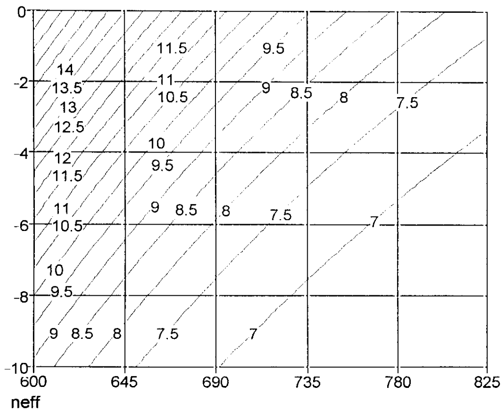
Fig.A.6.61. Representación tridimensional de n_{efectivo} , con respecto a la temperatura (K) y a la velocidad de deformación y mapa de representaciones de las curvas de nivel a n=cte .
