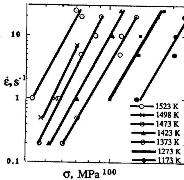
Fig.(15). Datos experimentales para el acero A3. \epsilon' (seg -1 ), \sigma (MPa).
