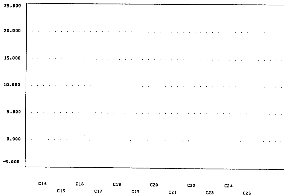
GRÁFICA 25. Representación "box-Cox" de las distribuciones de las variables correspondientes a las Gráficas 13,14,15,16,17,18,19,20,21,22,23,24
