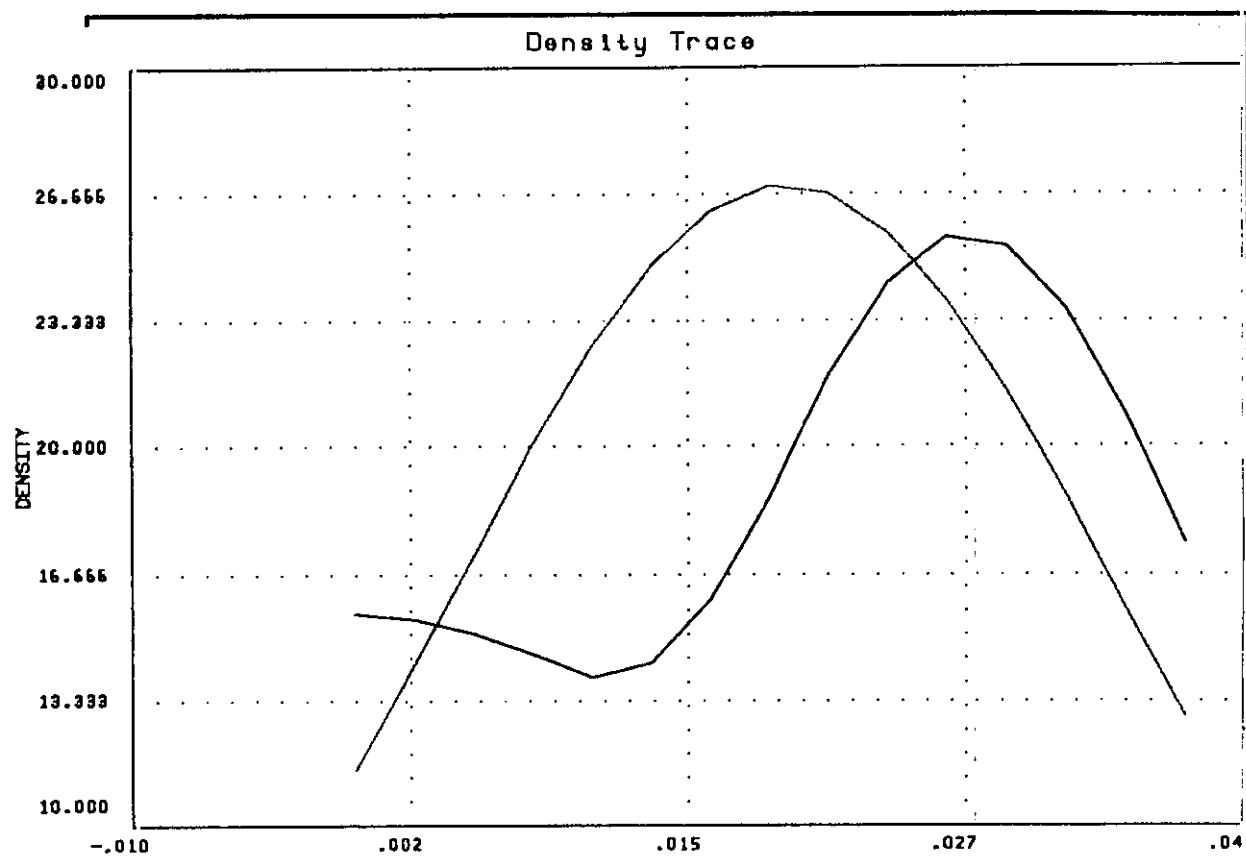
GRÁFICA 22. Representación de la función de densidad de la variable '% Al' de la tabla de datos
