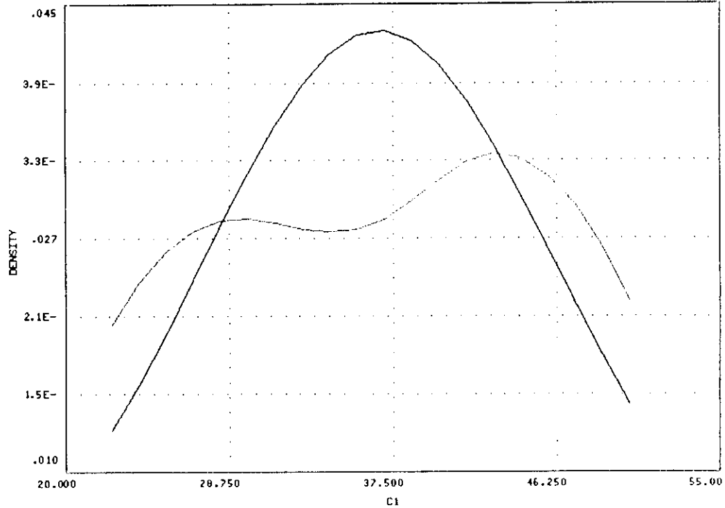
GRAFICA 1. Representación de de la función de densidad de la variable \ln(A) de la Tabla de datos 1. Comparada con la mejor distribución de densidad normal para los parámetros estadísticos representativos de la variable. \ln(A) presenta estructura bimodal.
