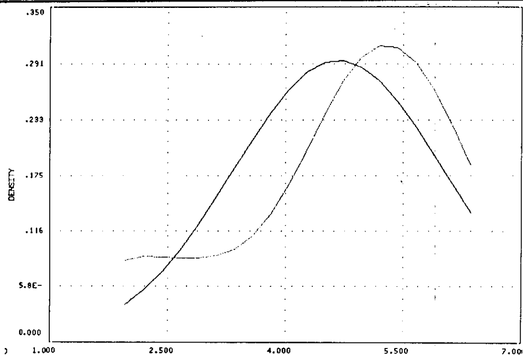
GRAFICA 1. Representación de la función de densidad de la variable n , de la Tabla de Datos 1. Comparada con la mejor distribución de densidad normal para los parámetros estadísticos representativos. Presenta una alta concentración y valores desagregados, con una incipiente bimodalidad.
