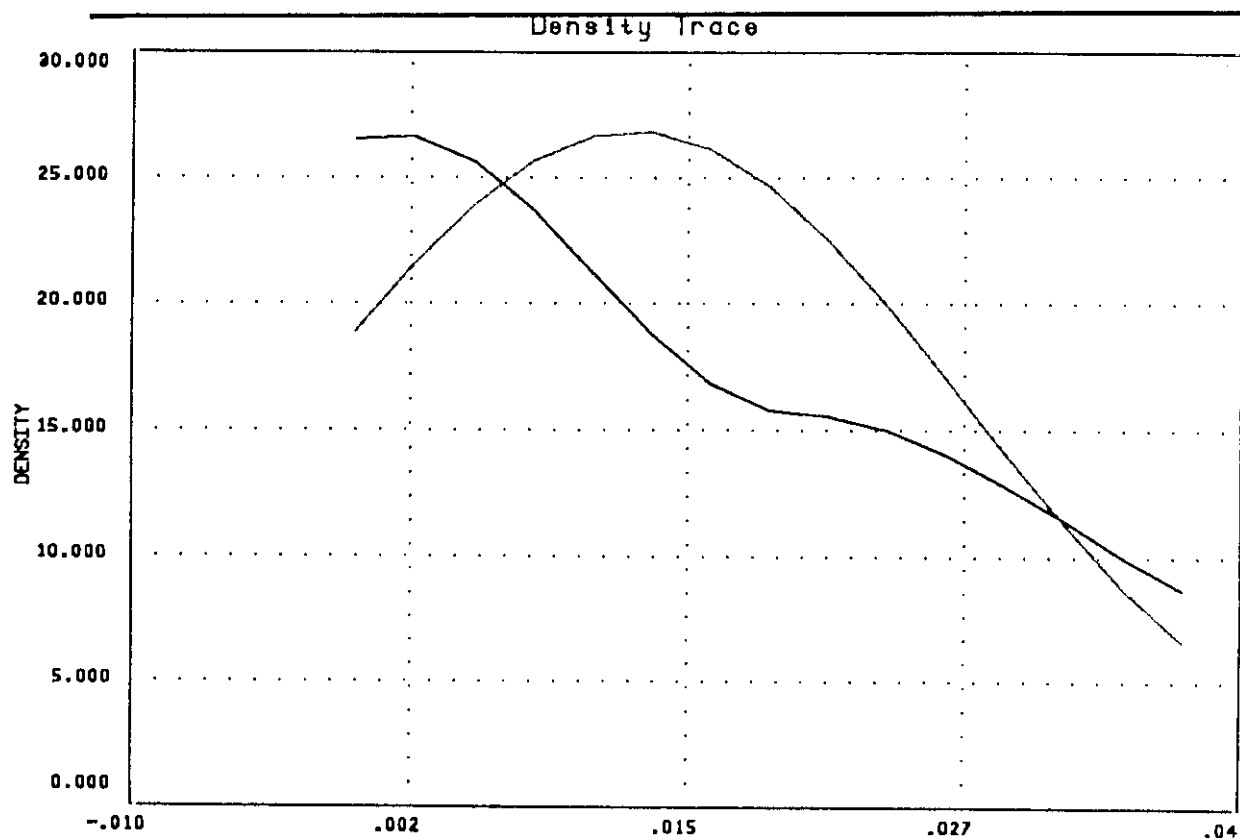
GRÁFICA 24. Representación de la función de densidad de la variable % TI de la tabla de datos
