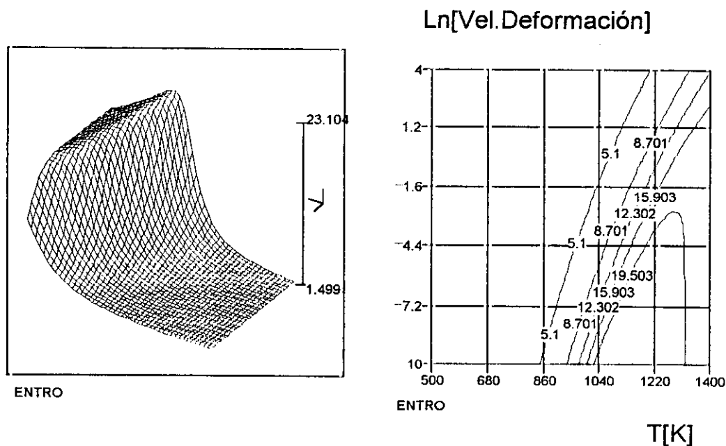
Fig.A.6.6. Representación diferencial del coeficiente de entropía \{s\} , frente a la temperatura y a la velocidad de deformación. Mapa de curvas de nivel. Isolineas son líneas de igual valor del coeficiente de entropía.
