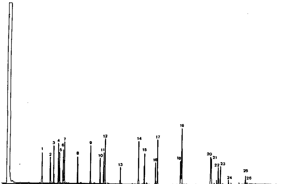
Cromatograma 2.- Fracción 2: Hidrocarburos aromáticos.
