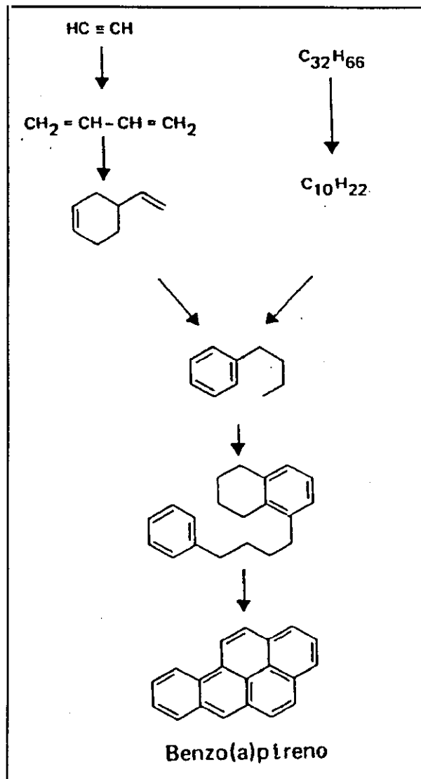
Figura 3.- Síntesis de Benzo(a)pireno según Badget (44).
