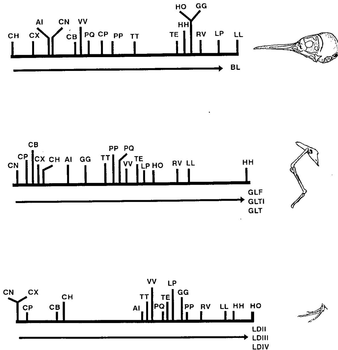
Fig. 3.- Situación de las especies a lo largo de los factores de tamaño. Abreviatura de las especies, AI: Arenaria interpres ; CB: Calidris alba ; CH: Charadrius hiaticula ; CN: Calidris minuta ; CP: Calidris alpina ; CX: Charadrius alexandrinus ; GG: Gallinago gallinago ; HH: Himantopus himantopus ; HO: Haematopus ostralegus ; LL: Limosa limosa ; LP: Limosa lapponica ; PP: Philomachus pugnax ; PQ: Pluvialis squatarola ; RV: Recurvirostra avosetta ; TE: Tringa erythropus ; TT: Tringa totanus ; VV: Vanellus vanellus .
