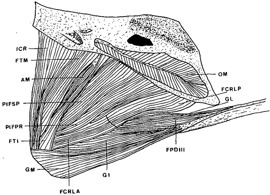
Fig. 21.- Vista medial de los músculos del muslo y de la pata.
