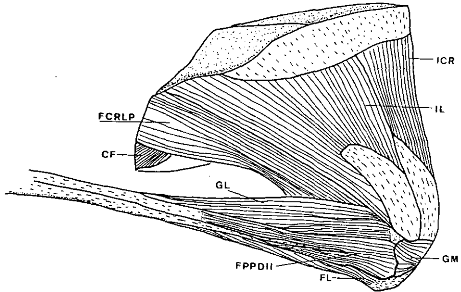
Fig. 18.- Vista lateral de la musculatura superficial del muslo y de la pata de Pluvialis squatarola . Abreviaturas de los músculos para las figuras 18-29: ABDII , abductor digiti II ; ABDIV , abductor digiti IV ; ADDII , adductor digiti II ; EBDIII , extensor brevis digiti III ; EBDIV , extensor brevis digiti IV ; CF , caudofemoralis ; EDL , extensor digitorum longus ; EHL , extensor hallucis longus ; FB , fibularis brevis ; FCRLA , flexor cruris lateralis pars accesoria ; FCRLP , flexor cruris lateralis pars pelvica ; FCRM , flexor cruris medialis ; FDL , flexor digitorum longus ; FHB , flexor hallucis brevis ; FHL , flexor hallucis longus ; FL , fibularis longus ; FPPDII , flexor perforatus digiti II ; FPPDIII , flexor perforatus digiti III ; FPPDIV , flexor perforatus digiti IV ; FPPDII , flexor perforatus et perforans digiti II ; FPPDIII , flexor perforatus et perforans digiti III ; FTED , femorotibialis externus pars distalis ; FTEP , femorotibialis externus pars proximalis ; FTI , femorotibialis internus ; FTM , femorotibialis medius ; GI , gastrocnemius pars intermedia ; GL , gastrocnemius pars lateralis ; GM , gastrocnemius pars medialis ; ICR , iliotibialis cranialis ; IF , iliofibularis ; IL , iliotibialis lateralis ; ITCA , iliotrochantericus caudalis ; ITCR , iliotrochantericus cranialis ; OM , obturatorius medialis ; PIFPR , puboischiofemoralis pars profundus ; PIFSP , puboischiofemoralis pars superficialis ; PL , plantaris ; PO , popliteus ; TCR , tibialis cranialis .
