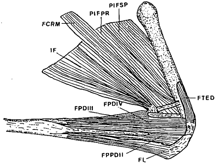
Fig. 23.- Vista lateral de los músculos profundos del muslo y superficiales de la pata.
