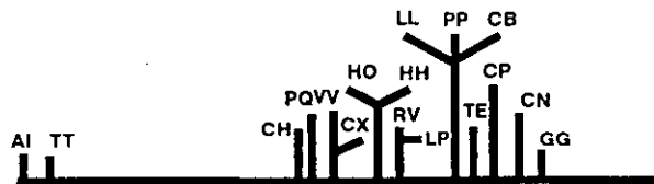
Fig. 38.- Situación de las especies en el gradiente definido por el 5º factor de comportamiento. Abreviaturas según figura 3.
