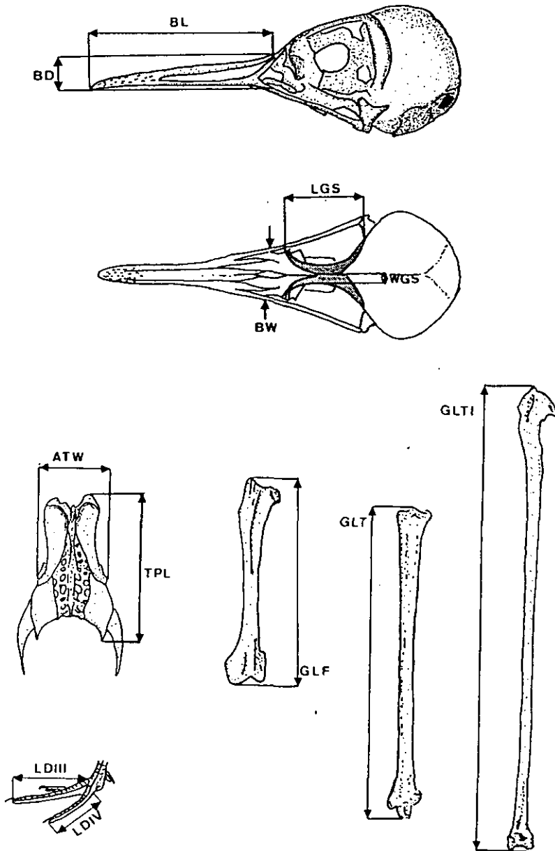
Fig. 1.- Medidas del cráneo y de las extremidades posteriores. ATW: anchura antitrocantérica; BD: altura del pico; BL: longitud del pico; BW: anchura del pico; GLF: longitud del fémur; GLT: longitud del tarsometatarso; GLTI: longitud del tibiotarso; LDIII: longitud del dedo III; LDIV: longitud del dedo IV; LGS: longitud de la glándula supraorbital; TPL: longitud total de la pelvis; WGS: anchura de la glándula supraorbital.
