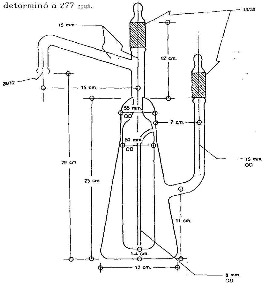
Figura 1.- Aparato utilizado para la destilación, en el análisis de furfurool.
