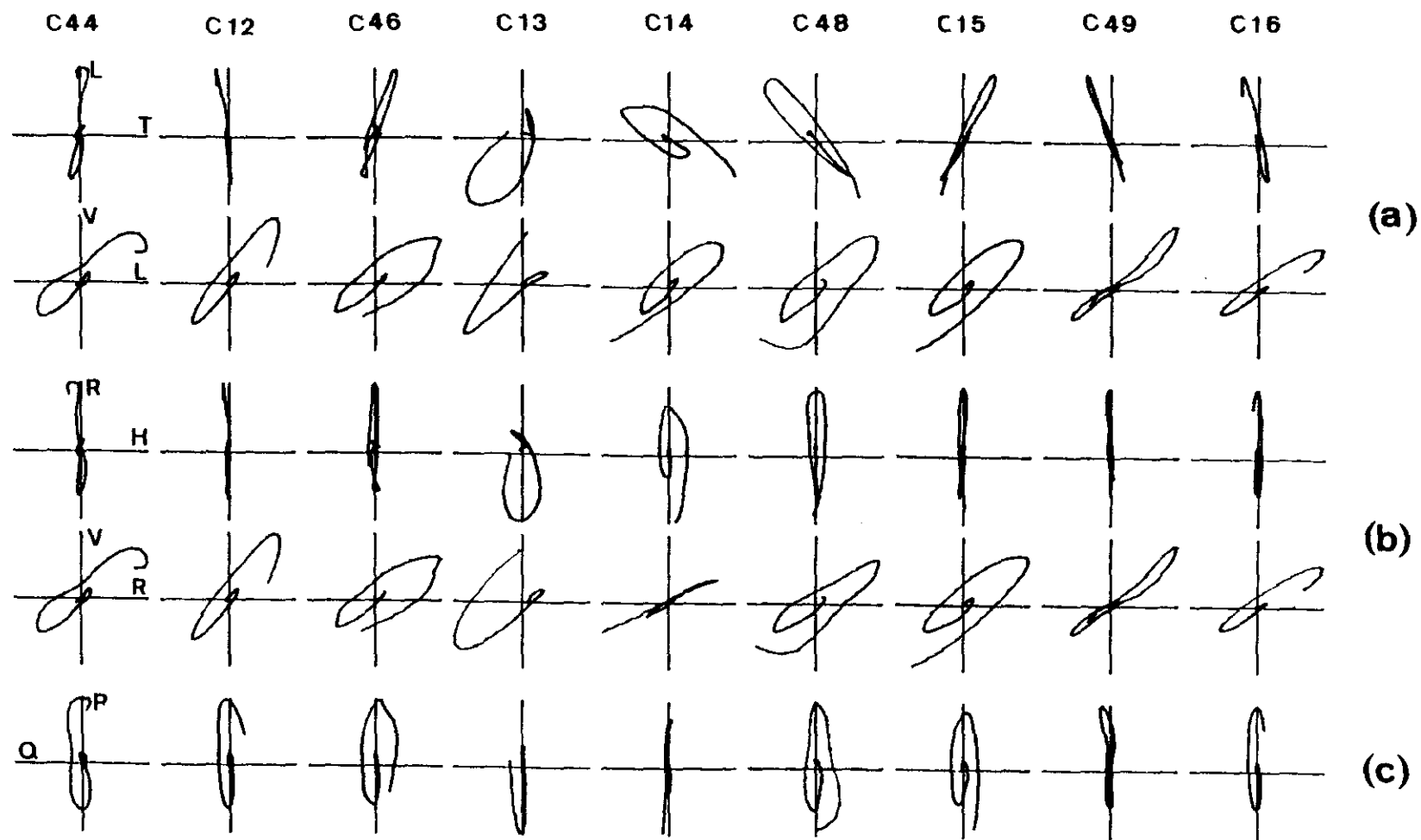
Figura 4.16. Diagramas del movimiento de la partícula de la fase P_g en los distintos sistemas de coordenadas referidos en el texto. (a) {T,L,V}; (b) {H,R,V}; (c) {H,Q,P}. Los números de la parte superior identifican los sismogramas (ver figura 4.15c).
