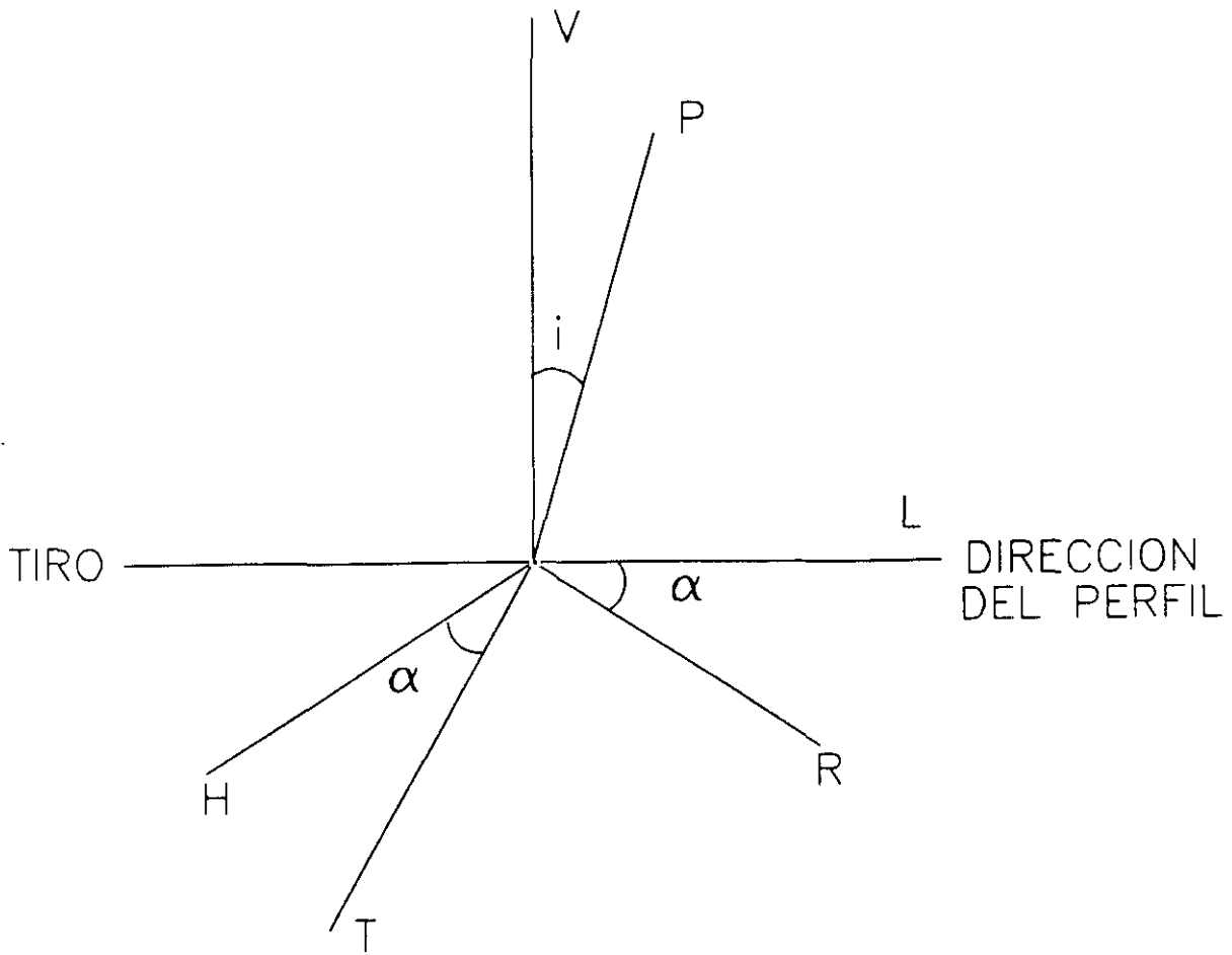
Figura 4.17. Relación geométrica entre los sistemas de ejes y ángulos de giro mencionados en el texto.
