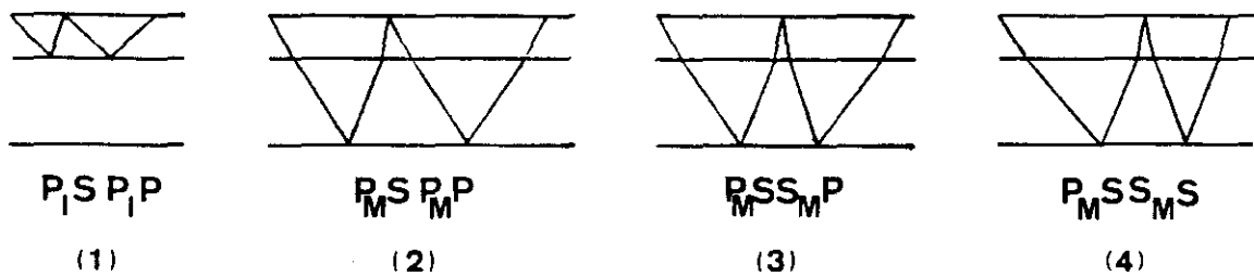
Figura 4.10. Sismogramas generados en la superficie libre del modelo de la Tabla 1. (a) Componente radial. Curvas de tiempo de recorrido y esquemas de identificación de las principales fases convertidas.
