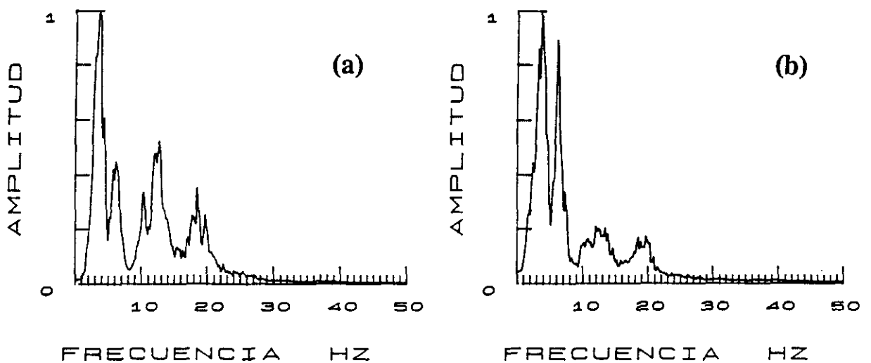
Figura 3.2. Espectros suma normalizados del perfil La Guardia-Ribadeo. (a) Espectro suma de las ondas P. (b) Espectro suma de las ondas S.
