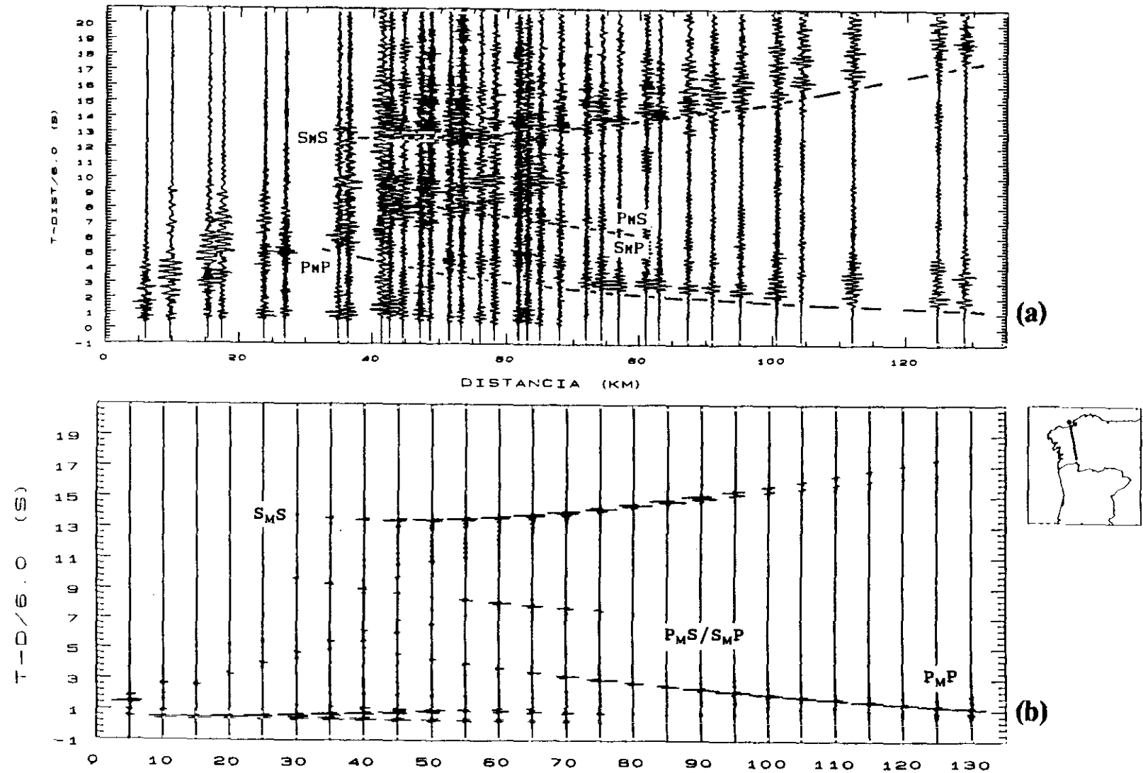
Figura 8.10(a) Ensamblaje completo de ondas P, S y convertidas, filtrado (1-15) Hz, para la componente radial del perfil La Coruña-La Cañiza, con las curvas de tiempo de recorrido de las fases P_M P y S_M S y convertidas en la Moho correlacionadas. (b) Componente radial de los sismogramas sintéticos calculados con el método de reflectividad para los modelos estructurales de velocidad P y S mostrados en el Apartado 7.4, supuestos homogéneos lateralmente.
