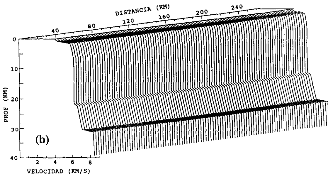
Figura 7.1.6(a). Modelo bidimensional de velocidad de ondas P para el perfil invertido La Guardia-Ribadeo. (b) Representación en perspectiva de la distribución V(z) , en la que se ha simplificado la corteza superior al eliminar la zona de alta velocidad.
