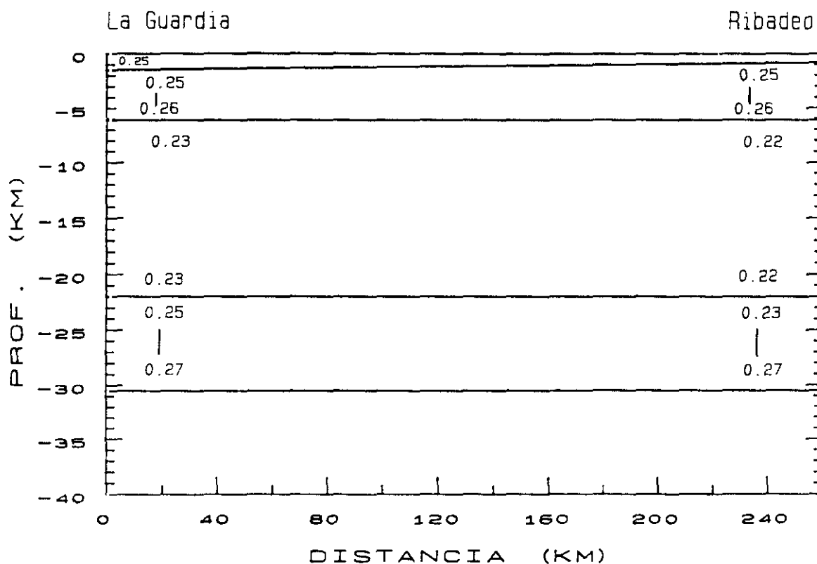
Figura 7.1.14. Modelo de la relación de Poisson, \sigma , para el perfil invertido Ribadeo-La Guardia.
