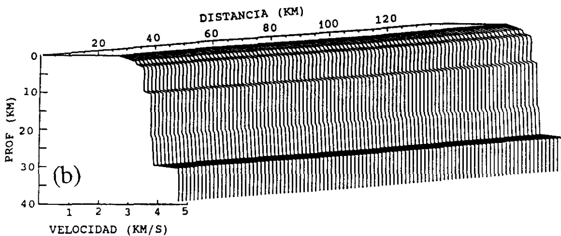
Figura 7.4.7(a) Modelo bidimensional de velocidad de ondas S para el perfil La Coruña-La Cañiza. (b) Representación en perspectiva de la distribución V_s(z) .
