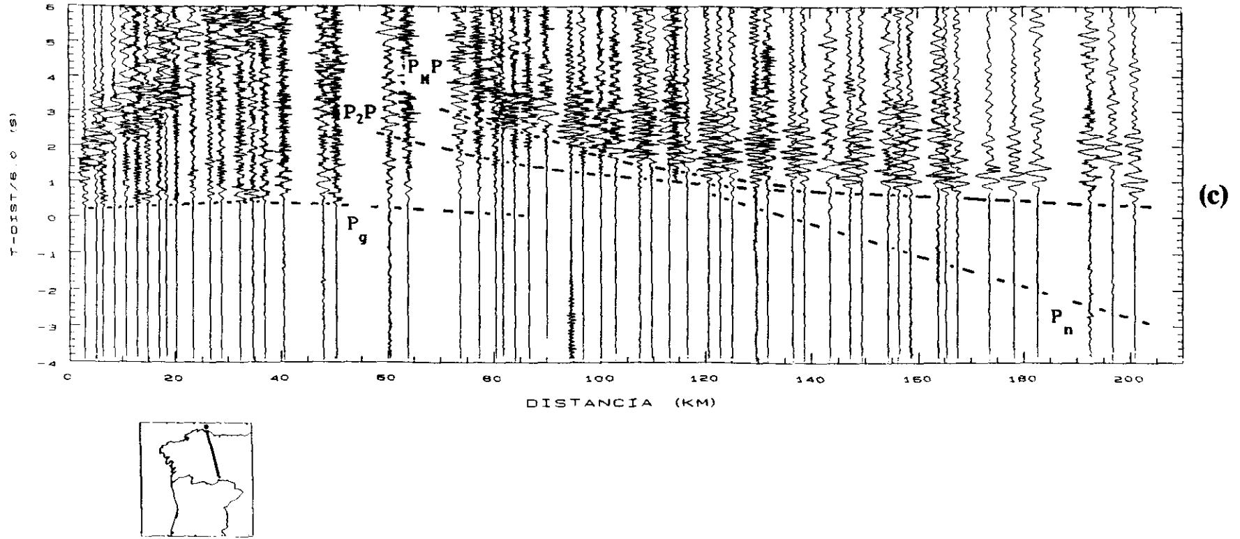
Figura 7.2.1. Ensamblajes de ondas P del perfil Vivero-Viana del Bollo. (a) Componente radial. (b) Componente transversal. (c) Componente vertical, con las curvas de tiempo de recorrido de las fases sísmicas correlacionadas.
