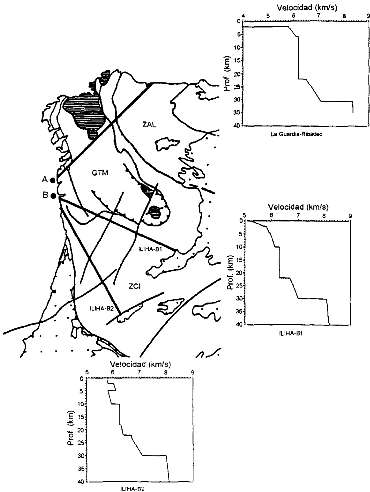
Figura 9.5 Variación acimutal de la estructura cortical en el noroeste de la Península Ibérica.
