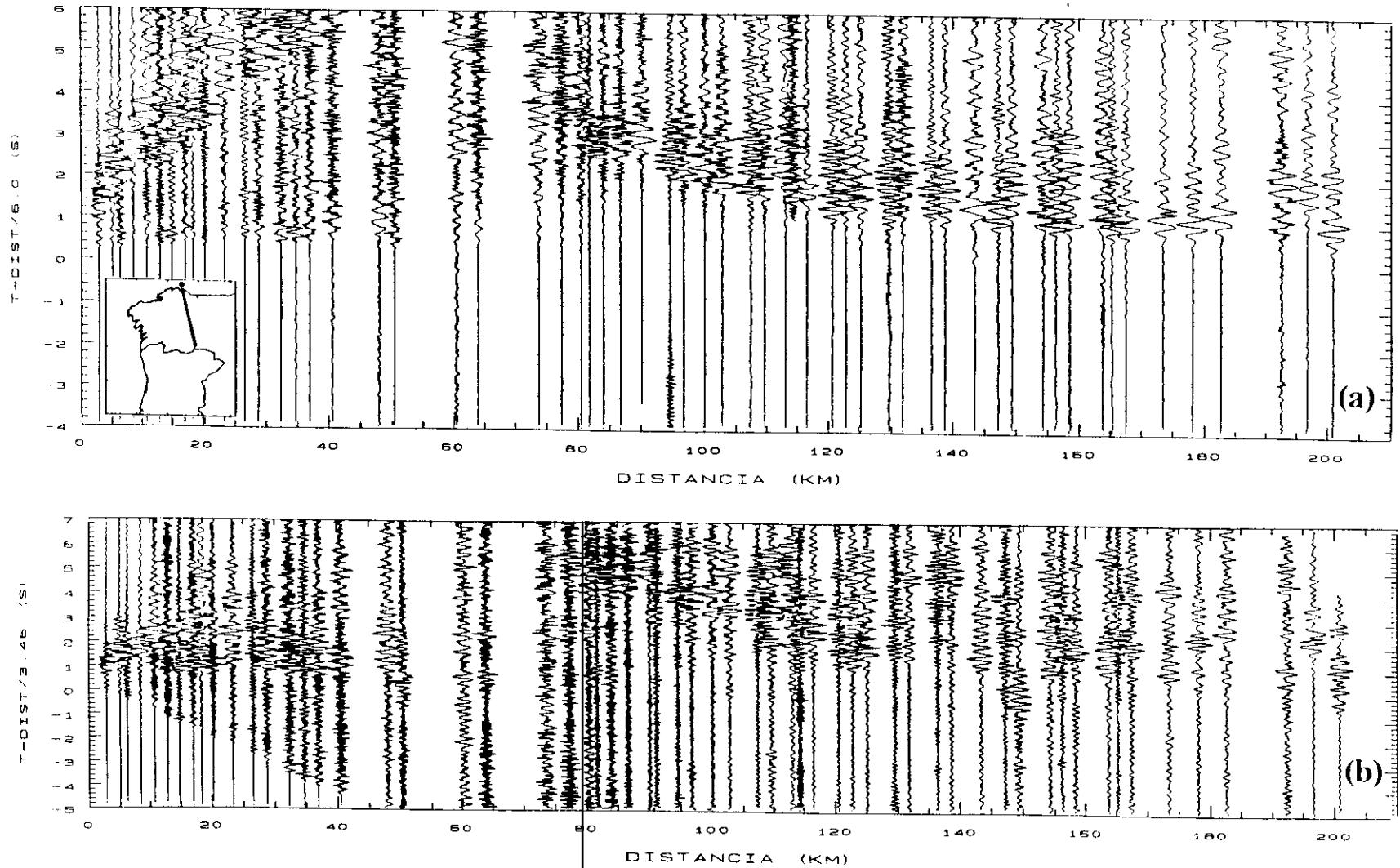
Figura 2.9. Perfil Vivero-Viana del Bollo. (a) Ensamblaje de ondas P, componente vertical. (b) Ensamblaje de ondas S, componente vertical.
