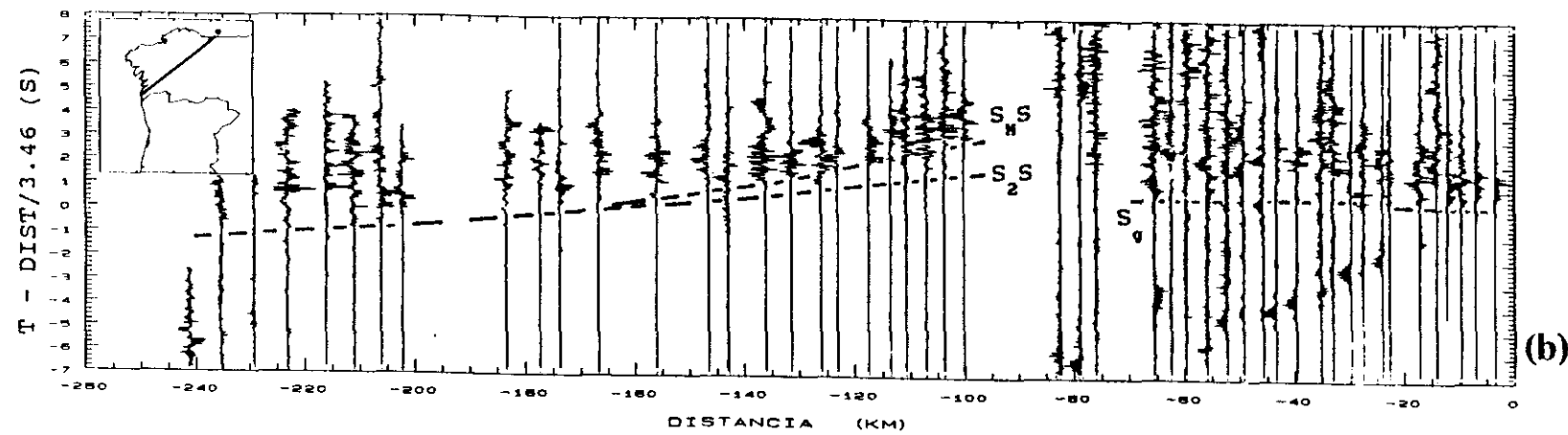
Figura 7.1.10. Ensamblaje de ondas S del perfil Ribadeo-La Guardia, con las curvas de tiempo de recorrido de las fases sísmicas correlacionadas. (a) Componente radial, filtrada (1-10) Hz. (b) Ensamblaje producto de las componentes radial y vertical.
