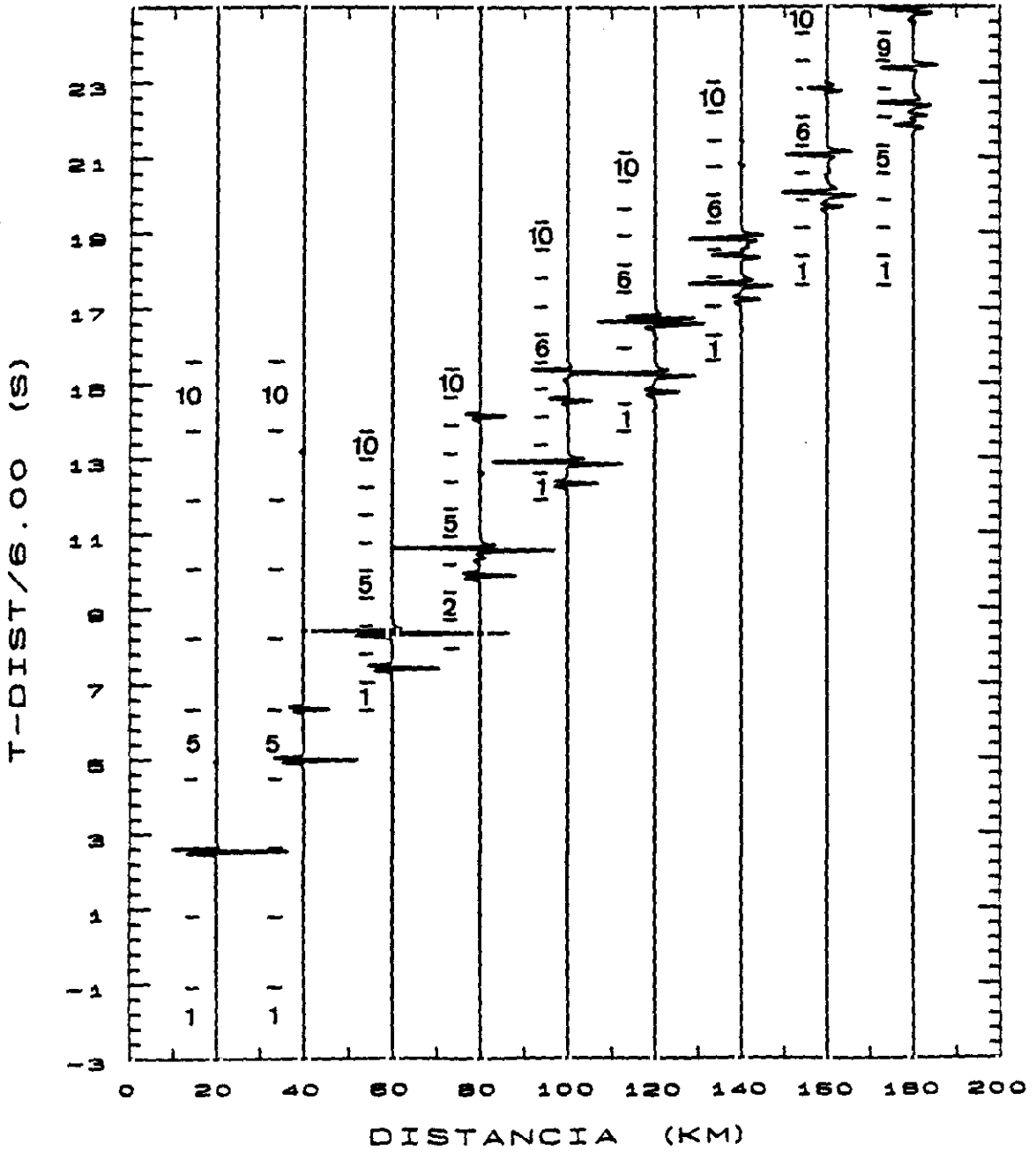
Figura 4.3(c). Componente transversal. Los números a la izquierda de los sismogramas identifican las ventanas de tiempo utilizadas para construir los diagramas de polarización de la figura 4.5.
