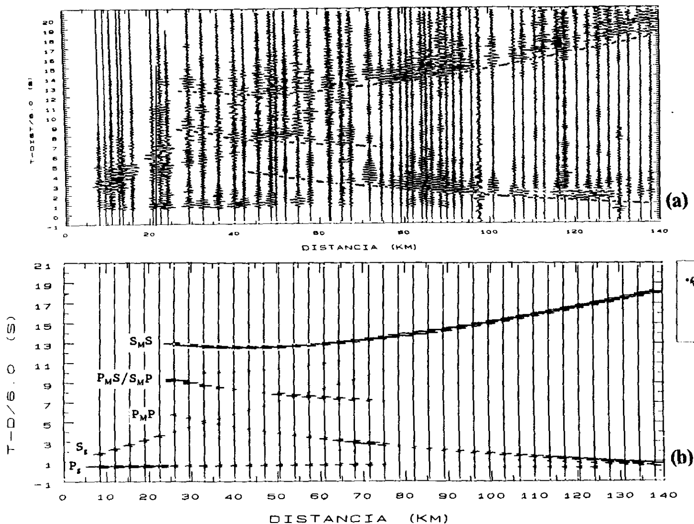
Figura 8.9(a) Ensamblaje completo de ondas P, S y convertidas, filtrado (1-15) Hz, para la componente radial del perfil Finisterre-Sarria, con las curvas de tiempo de recorrido de las fases P_M P y S_M S y convertidas en la Moho correlacionadas. (b) Componente radial de los sismogramas sintéticos calculados a partir de los modelos estructurales de velocidad P y S mostrados en el Apartado 7.3.
