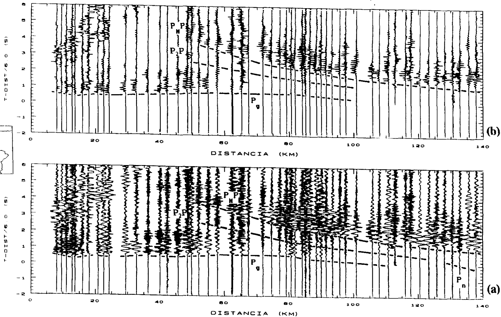
Figura 7.3.7. Perfil Finisterre-Sarria. (a) Ensamblaje de ondas P, para la componente vertical. (b) Ensamblaje producto de las componentes radial y vertical de los sismogramas. Las líneas dibujadas indican las curvas de tiempo de recorrido de las fases sísmicas correlacionadas.
