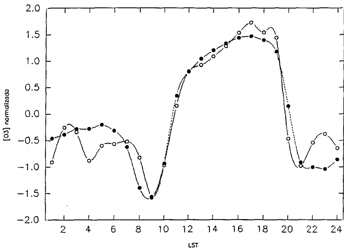
Fig 4.16 Evolución diaria de las concentraciones de ozono; o día 27-12-91; ● día medio de invierno.
