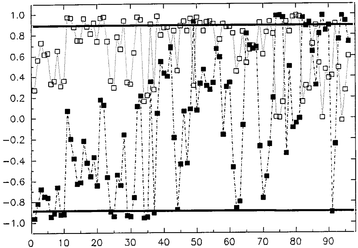
Fig 4.26. Correlaciones entre los vectores propios y los vectores distancia de la serie de primavera; \square respecto al autovector P_1 ; \blacksquare respecto al autovector P_2 .
