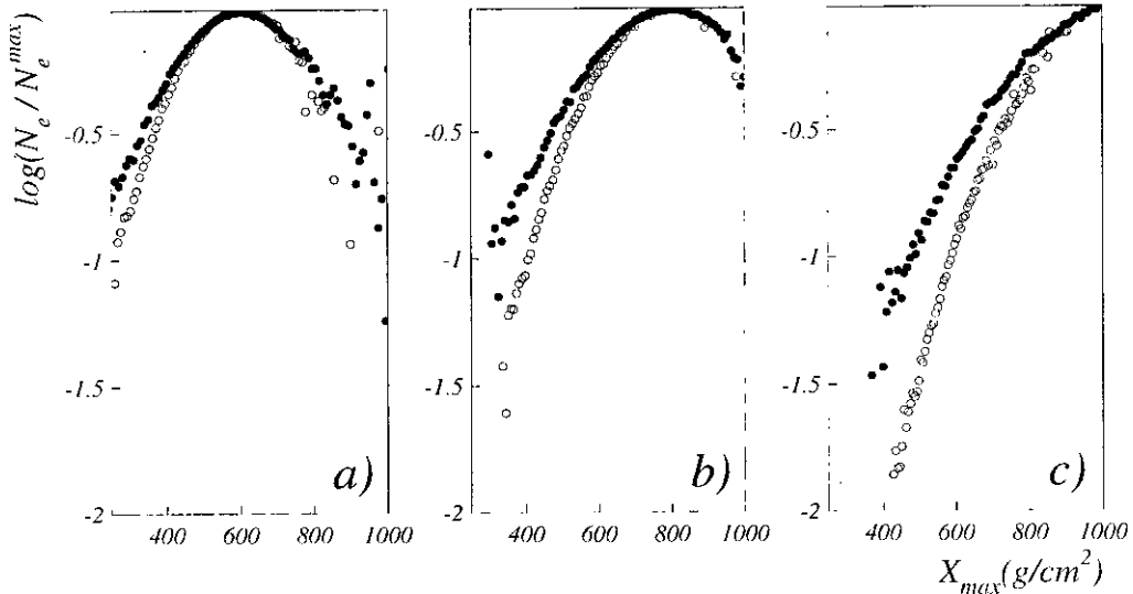
Figura 4.8: Número de electrones en tierra sobre número de electrones en el máximo de la cascada frente a la profundidad de máximo desarrollo como se espera a niveles de observación de 600 \text{ g/cm}^2 (a), 800 \text{ g/cm}^2 (b) y nivel del mar (c). Las partículas primarias son protones (puntos negros) y rayos \gamma (puntos blancos) en los rangos de energía de 1-10^2 \text{ TeV} (a), 10-10^3 (b) y 10^2 - 10^4 \text{ TeV} (c). Cada punto representa el valor medio de la distribución de valores de N_e/N_e^{max} para los eventos para un correspondiente valor de X_{max} .
