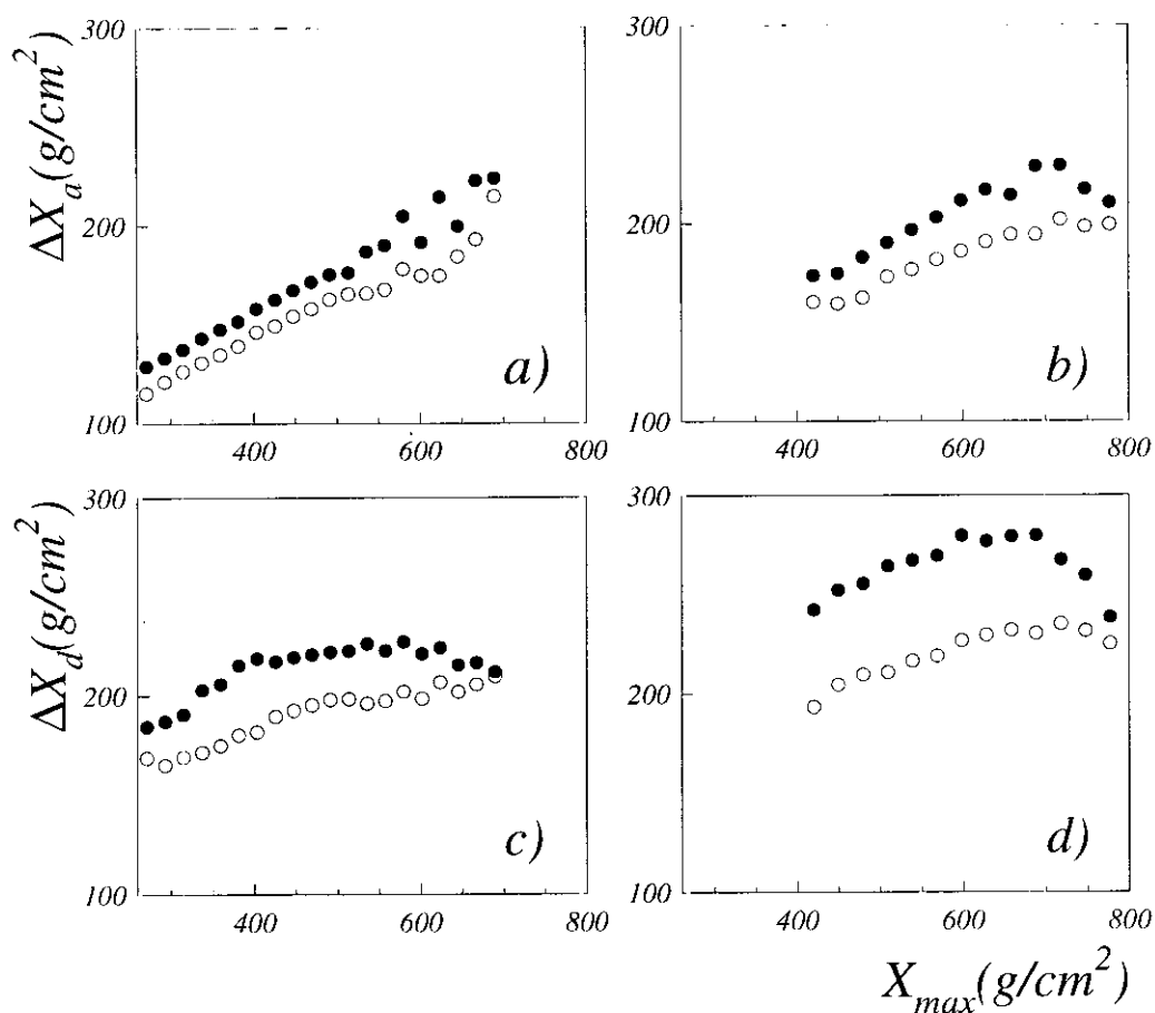
Figura 4.16: Semianchura antes del máximo (a,b) y más allá del máximo (c,d) del desarrollo longitudinal frente a la profundidad del máximo de la cascada para cascadas iniciadas por protones (círculos negros) y rayos-gamma (círculos blancos) en el rango de energía de 1 – 100 TeV (a,c) y 10^2 - 10^4 TeV (b,d). Cada punto representa el valor medio de la semianchura de la distribución para todos los eventos correspondientes a un valor de X_{max} .
