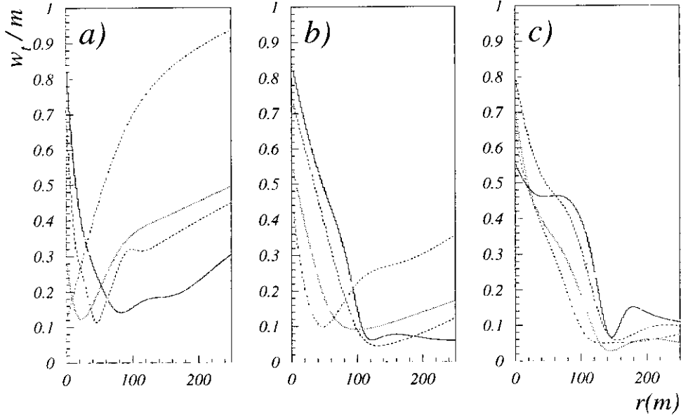
Figura 4.7: Anchura total de las fluctuaciones de la distribución radial de luz Cherenkov dividida por el valor medio, a tres niveles de observación: 600 \text{ g/cm}^2 (a), 800 \text{ g/cm}^2 (b) y nivel del mar (c). Las energías correspondientes son 10 TeV (línea continua), 100 TeV (línea quebrada), 1000 TeV (línea punteada) y 10^4 TeV (línea mixta, puntos y rectas). Las curvas representan una suavización de los resultados obtenidos.
