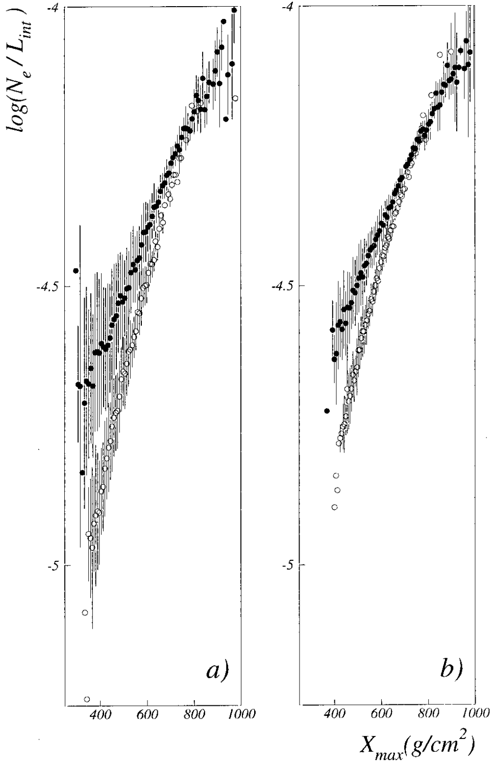
Figura 4.10: Lo mismo que en la figura 4.9 a 800 \text{ g/cm}^2 y para rangos de energía (para rayos \gamma ) de 10-100 TeV (a) y 100-1000 TeV (b).
