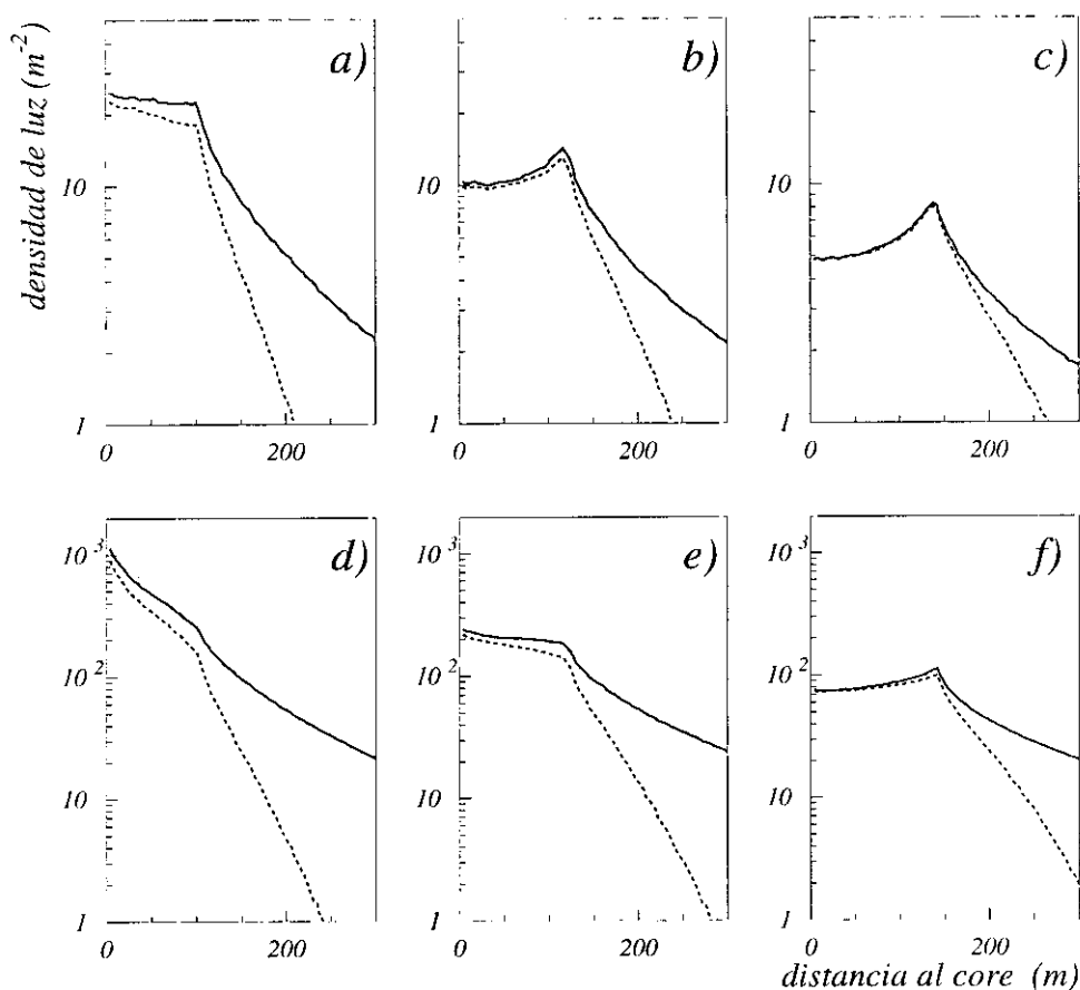
Figura 3.7: Distribución lateral de todos los fotones Cherenkov (curva continua) y de los que tienen un ángulo zenital menor que 1.4 grados (línea quebrada) para cascadas \gamma con incidencia vertical de 0.1 TeV a: a) 600 \text{g}/\text{cm}^2 ; b) 800 \text{g}/\text{cm}^2 ;y c) nivel del mar; y de 1TeV a: d) 600 \text{g}/\text{cm}^2 ; e) 800 \text{g}/\text{cm}^2 ;y f) nivel del mar.
