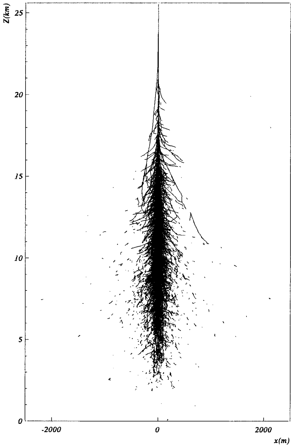
Figura 2.2: Cascada atmosférica de e^\pm iniciada por un rayo \gamma en incidencia vertical y con 300 GeV de energía.
