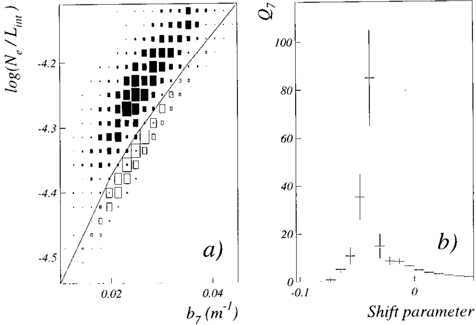
Figura 4.19: a) N_e/L_{int} frente a b_7 para el intervalo de energía de 10 – 10 2 TeV a una profundidad de observación de 600 g/cm 2 . El tamaño de las cajas es proporcional al logaritmo del número de eventos. Las cajas negras (blancas) corresponden a cascadas iniciadas por protones (gammas). b) El factor de calidad frente al desplazamiento vertical respecto de la línea de corte mostrada en a).
