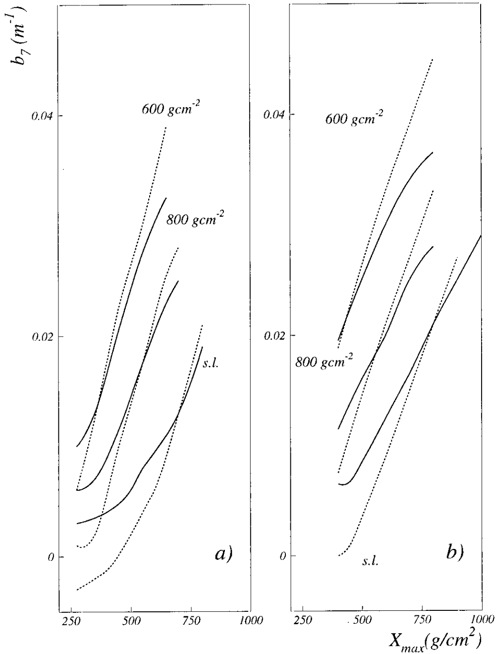
Figura 4.15: Pendiente de la distribución radial de luz Cherenkov en tierra frente a X_{max} para cascadas iniciadas por protones (línea continua) y rayos \gamma (línea discontinua). Las profundidades de observación son 600 g/cm^2 , 800 g/cm^2 y nivel del mar (s.l.). Los rangos de energía para rayos \gamma son 1 – 10 2 TeV (a) y 10 2 – 10 4 (b). Las líneas representan una suavización de las medias de las distribuciones correspondientes.
